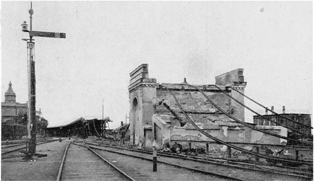
Une des constructions en briques sur lesquelles passait la voie terrée desservant les quais et les môle.
