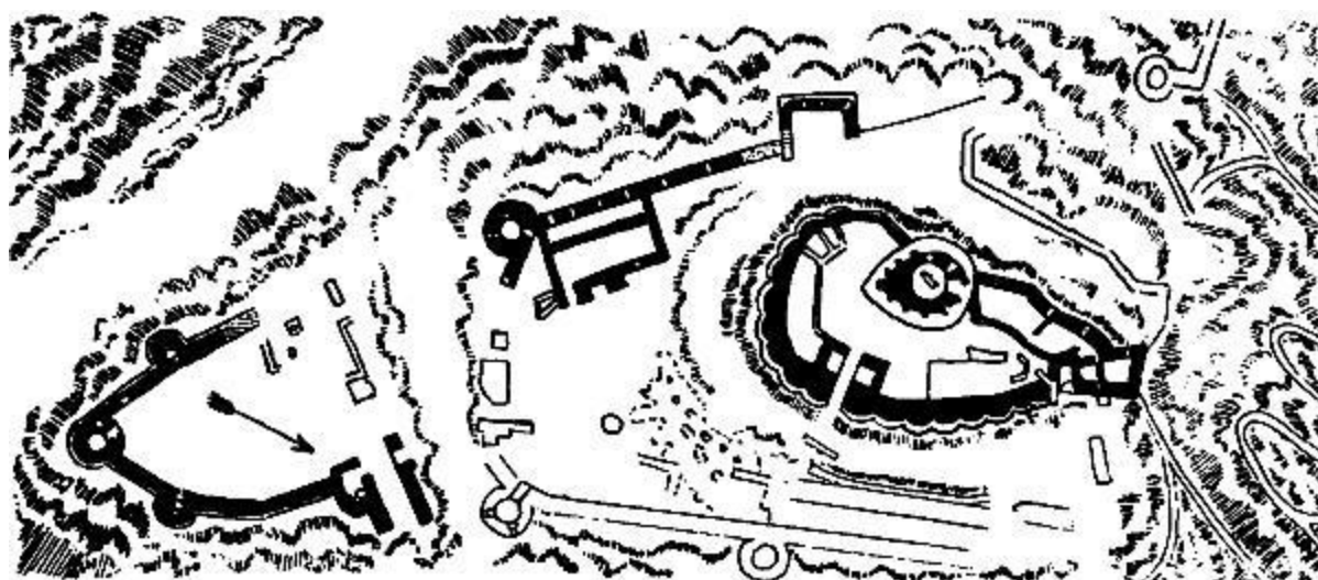
Château-Gaillard; Plan
