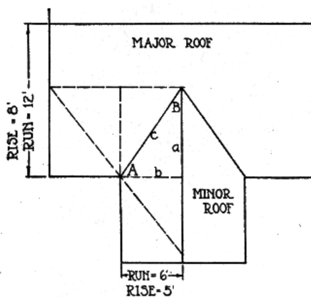
Fig. 88-a. Uneven Pitches
