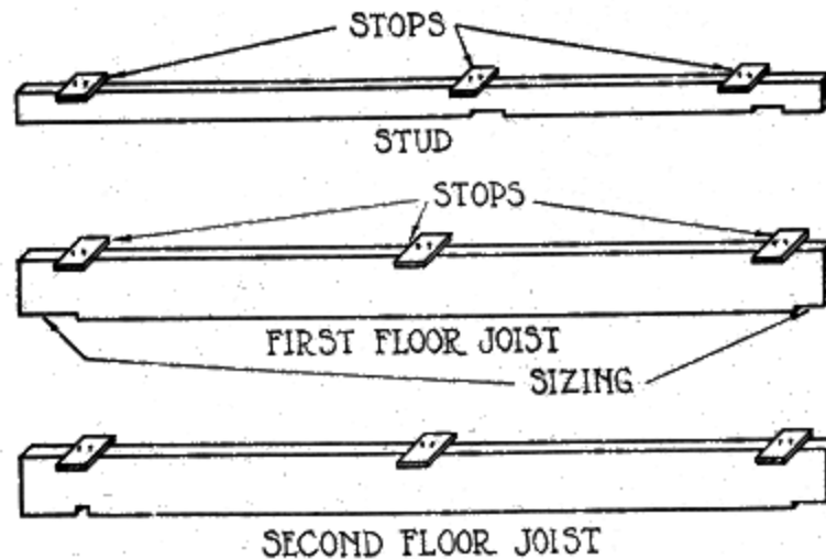
Fig. 30. Stud and Joist Patterns
