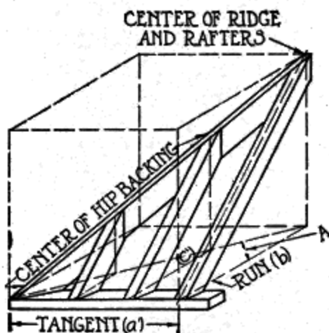
Fig. 58-a. Hip Rafter.
