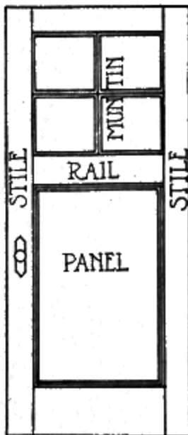
Fig. 132. Door Parts
