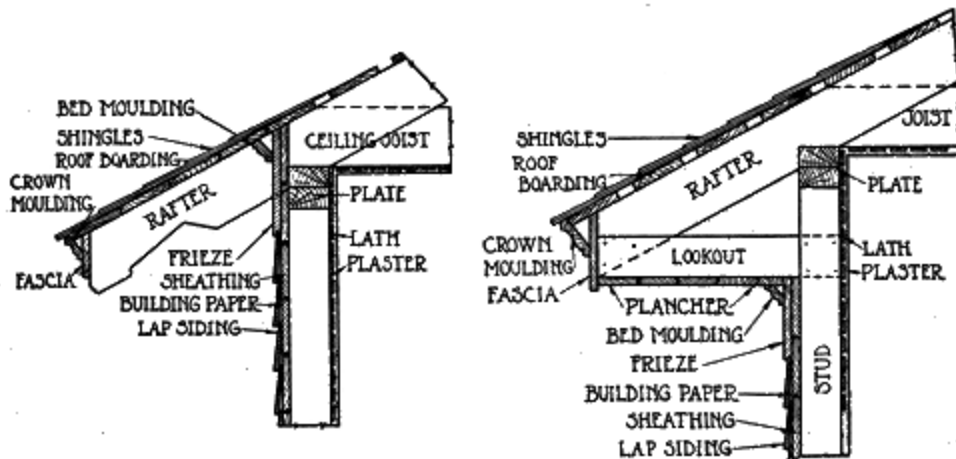
Fig. 95. Skeleton Cornice Fig. 96. Box Cornice
