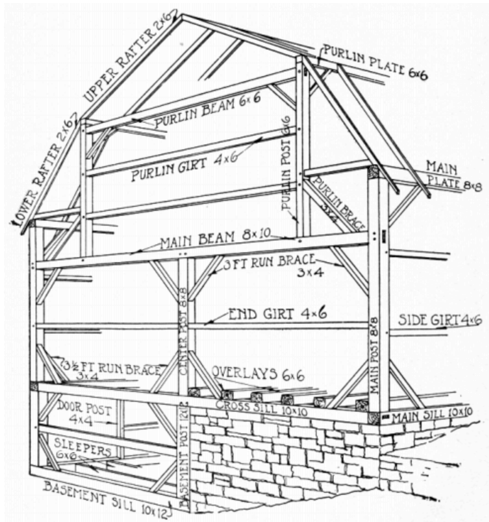
Fig. 17. Heavy Timber Barn
