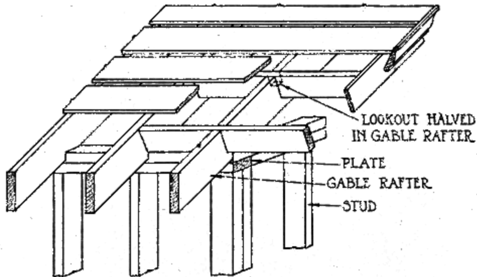
Fig. 97-a. Skeleton Cornice
