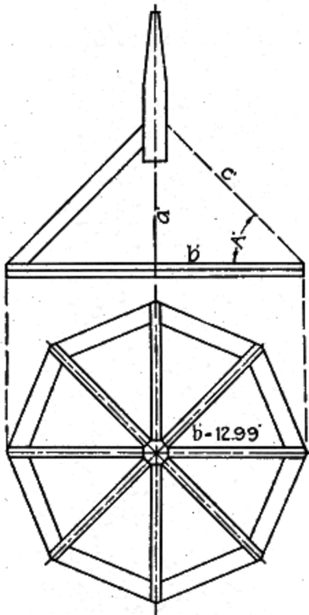
Fig. 76. King-Post
