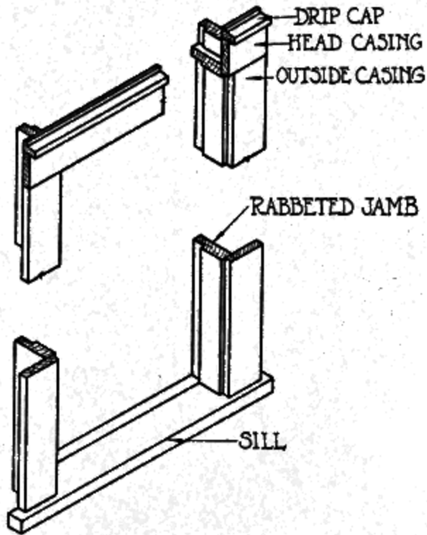
Fig. 145. Detail of Door Frame
