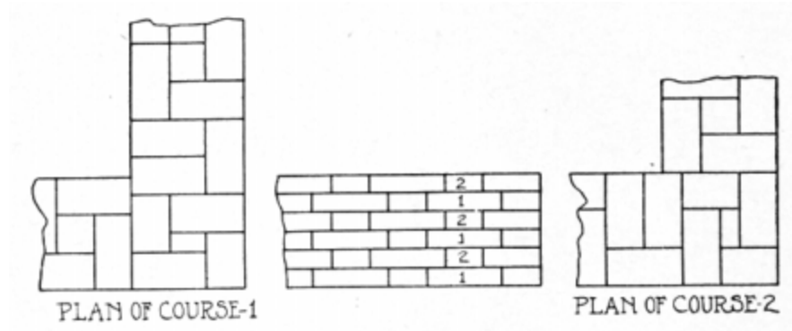
Fig. 10. Flemish Bond
