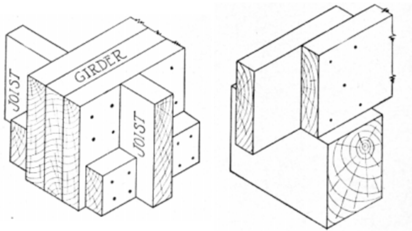
Fig. 22-a Fig. 22-b. Girder Types
