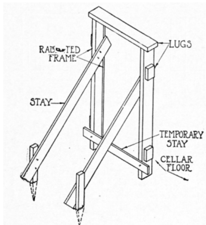
Fig. 14. Basement Door Frame
