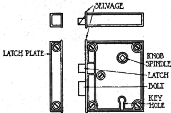
Fig. 140. Rim Lock
