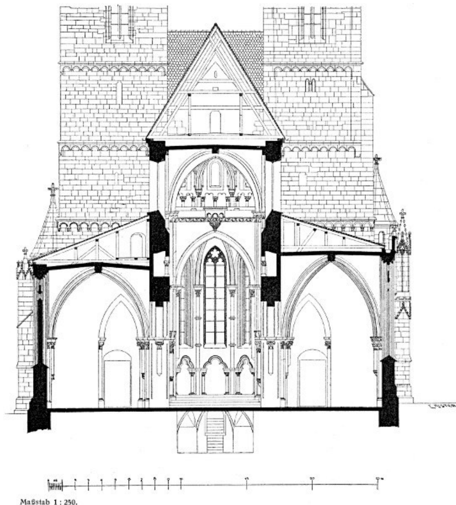
Abb. 19. Querschnitt durch das Mittelschiff und die Seitenschiffe.
