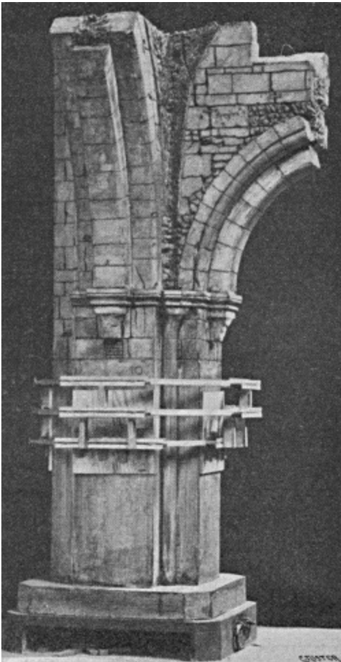
Abb. 44. Modell eines zum Teil armierten Vitrumspfeilers.
