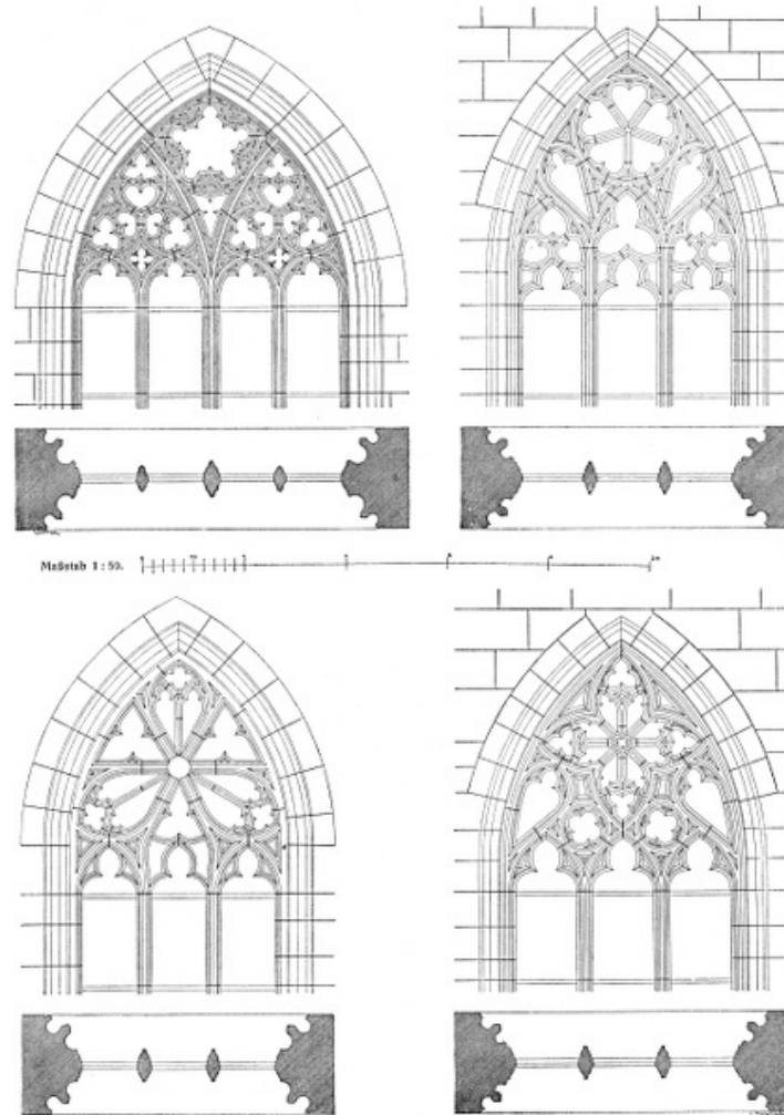
Abb. 21 a–d. Fenster-Maßwerke der Seitenschiffe.
