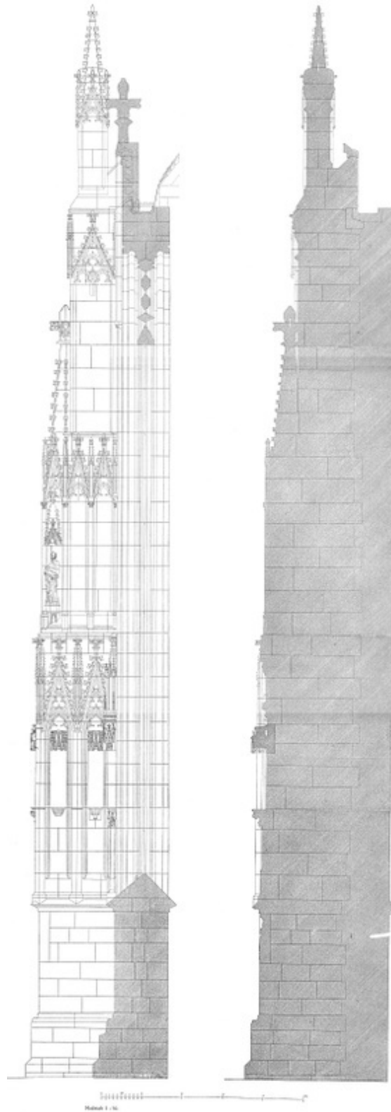
Seitenansicht und Schnitt eines Strebe Pfeilers am Ostchor.
