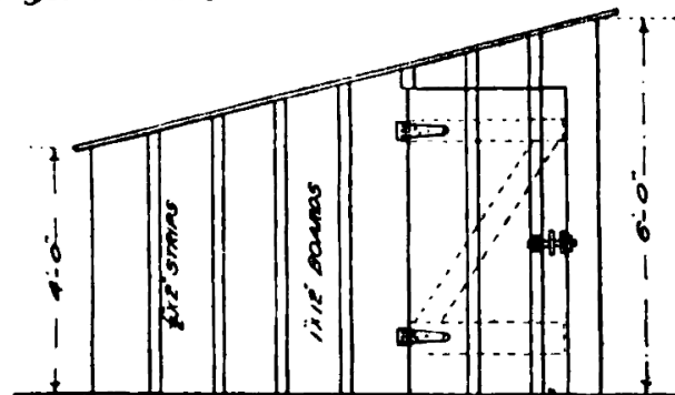
END ELEVATION
