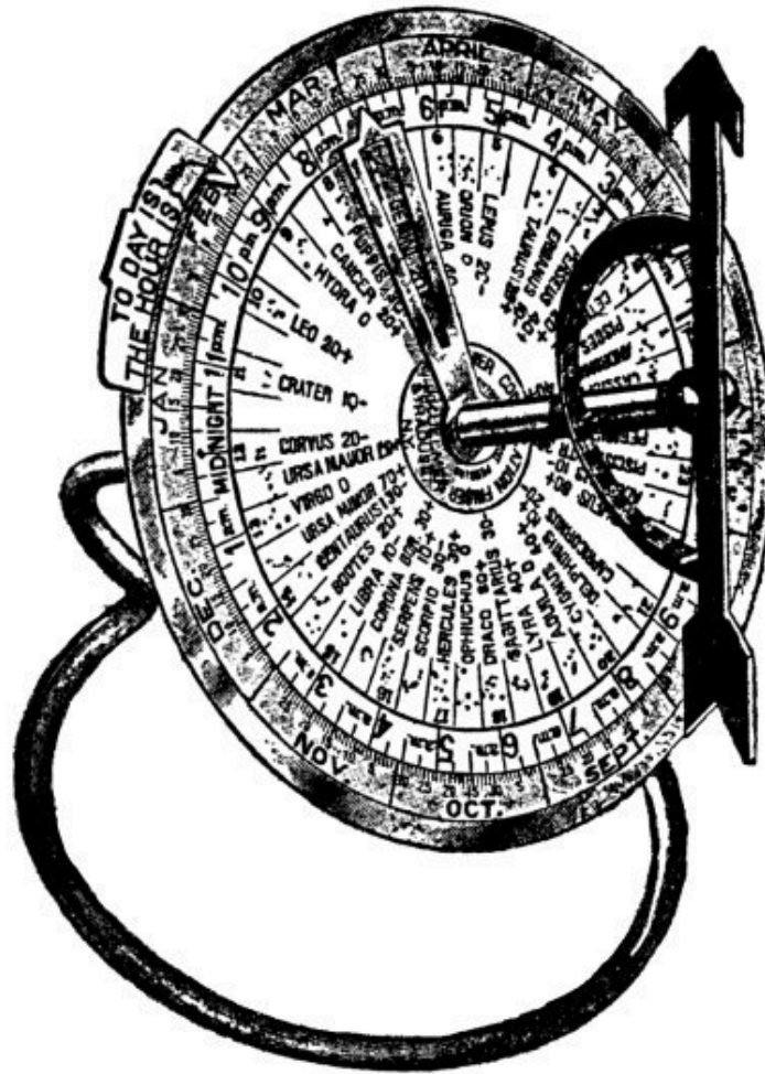
FIG. 186.—KULLMER STAR FINDER.
