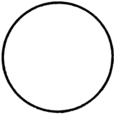
FIG. 58.—URANUS.
