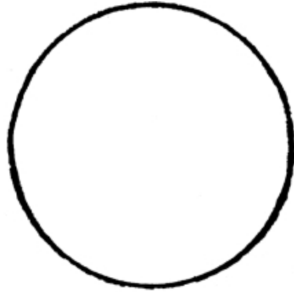
FIG. 59.—NEPTUNE.
