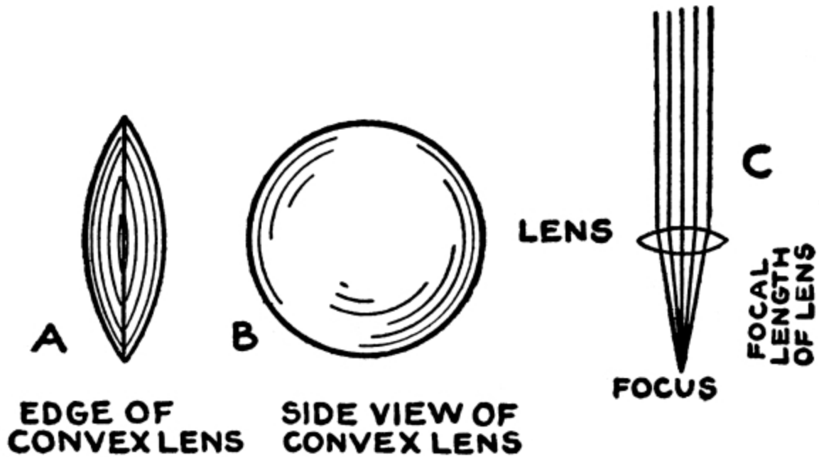
FIG. 146.—CONVEX LENS.
