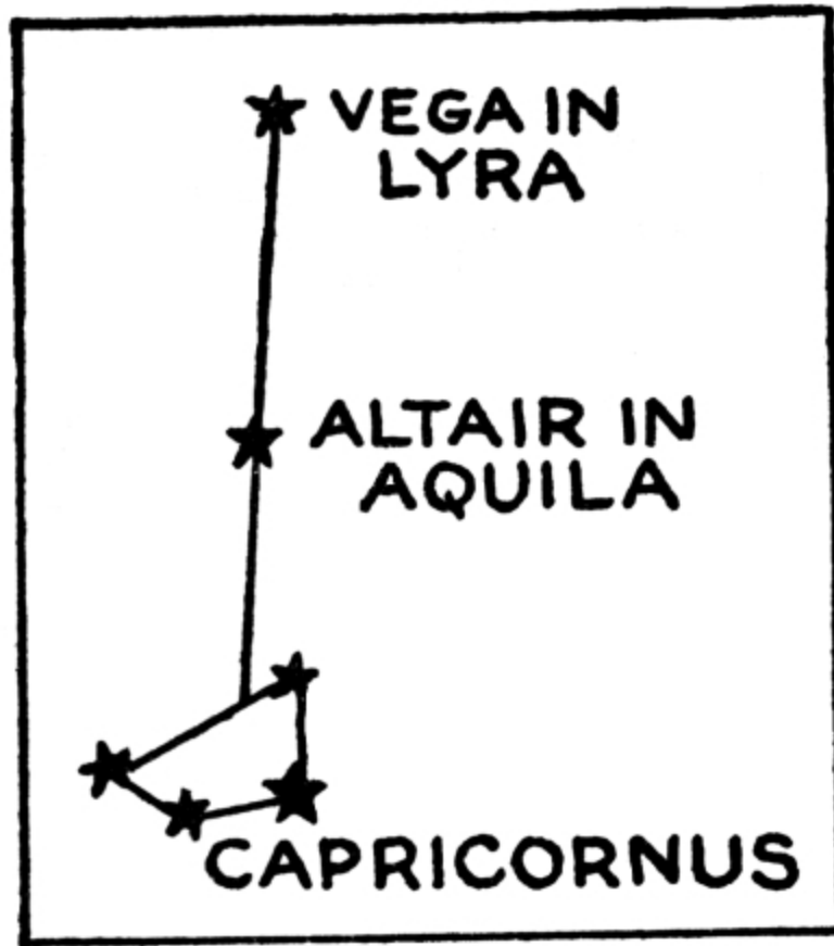
FIG. 179.—LYRA, AQUILA, CAPRICORNUS.
