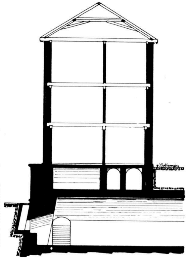
Durchschnitt im südwestlichen Flügel
