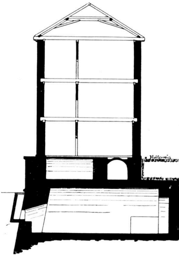
Durchschnitt im nordöstlichen Flügel
