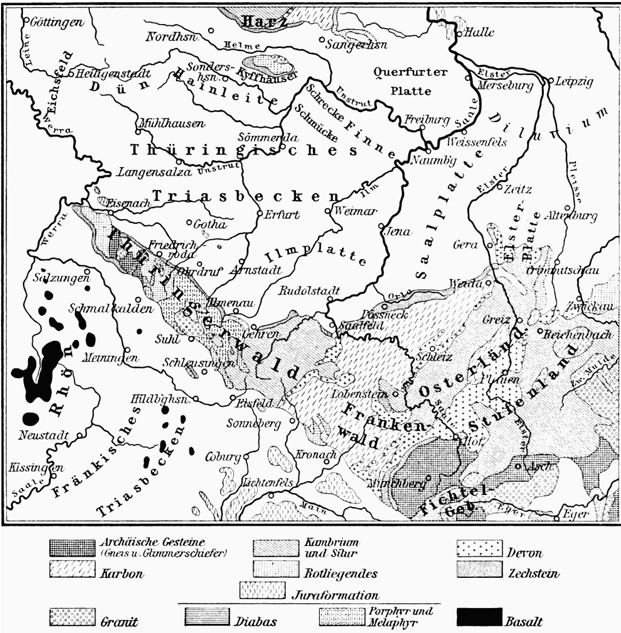
Abb. 4. Geologische Skizze von Thüringen.
