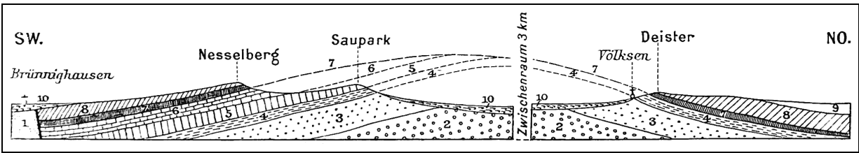
Abb. 6. Der Deister-Saupark-Sattel. (Zu Seite 9 u. 18 .)
