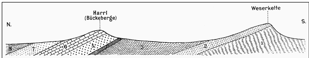
Abb. 4. Profil durch Weserkette und Bückeberge.
