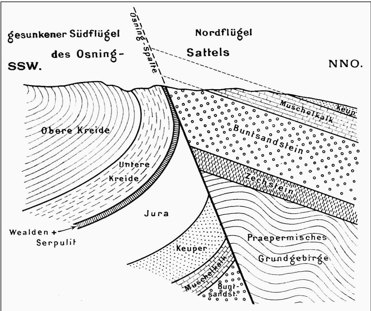
Abb. 10. Schematisches Profil des Osnings (unter Fortlassung der Zwischenstaffeln zwischen Kreide und Buntsandstein).
