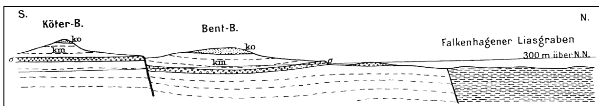
Abb. 14. Profil durch Falkenhagener Liasgraben und Köterberg. Maßstab 1 : 40000. (Zu Seite 18. )
