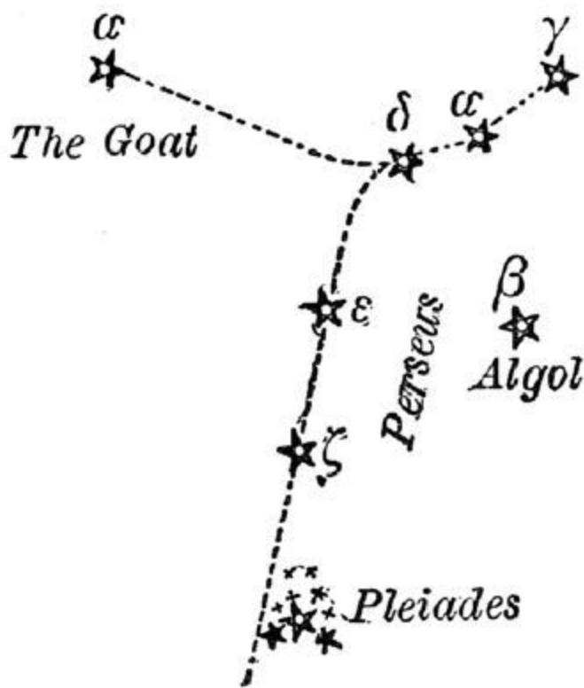
FIG. 7.—Perseus, the Pleiades, Capella.
