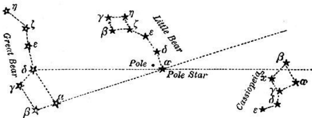
FIG. 5.—To find Cassiopeia.
