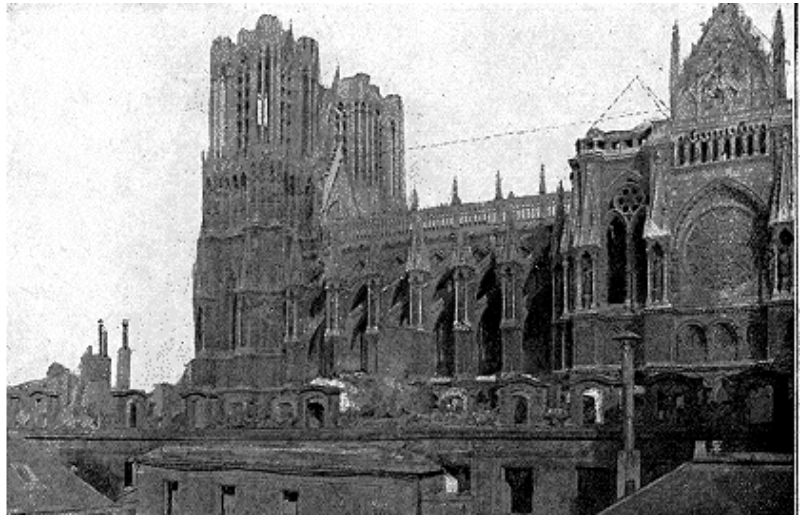
La façade méridionale de Notre-Dame de Reims après l'incendie. Les lignes pointillées indiquent les profils des toitures détruites.
