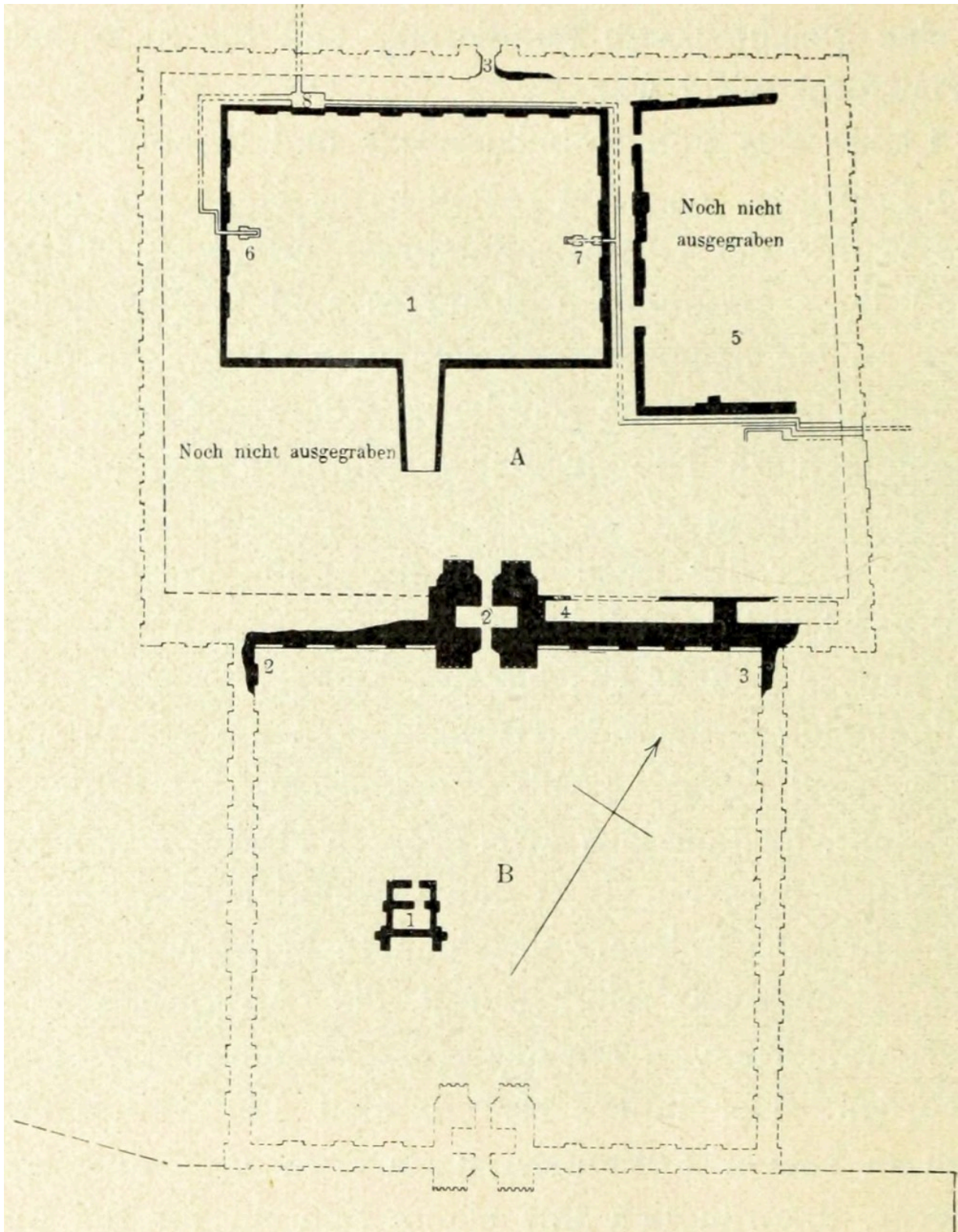
Abb. 27. Grundplan des Bêl-Tempels zu Nippur. Rekonstruiert von Hilprecht, gezeichnet von Fisher.
