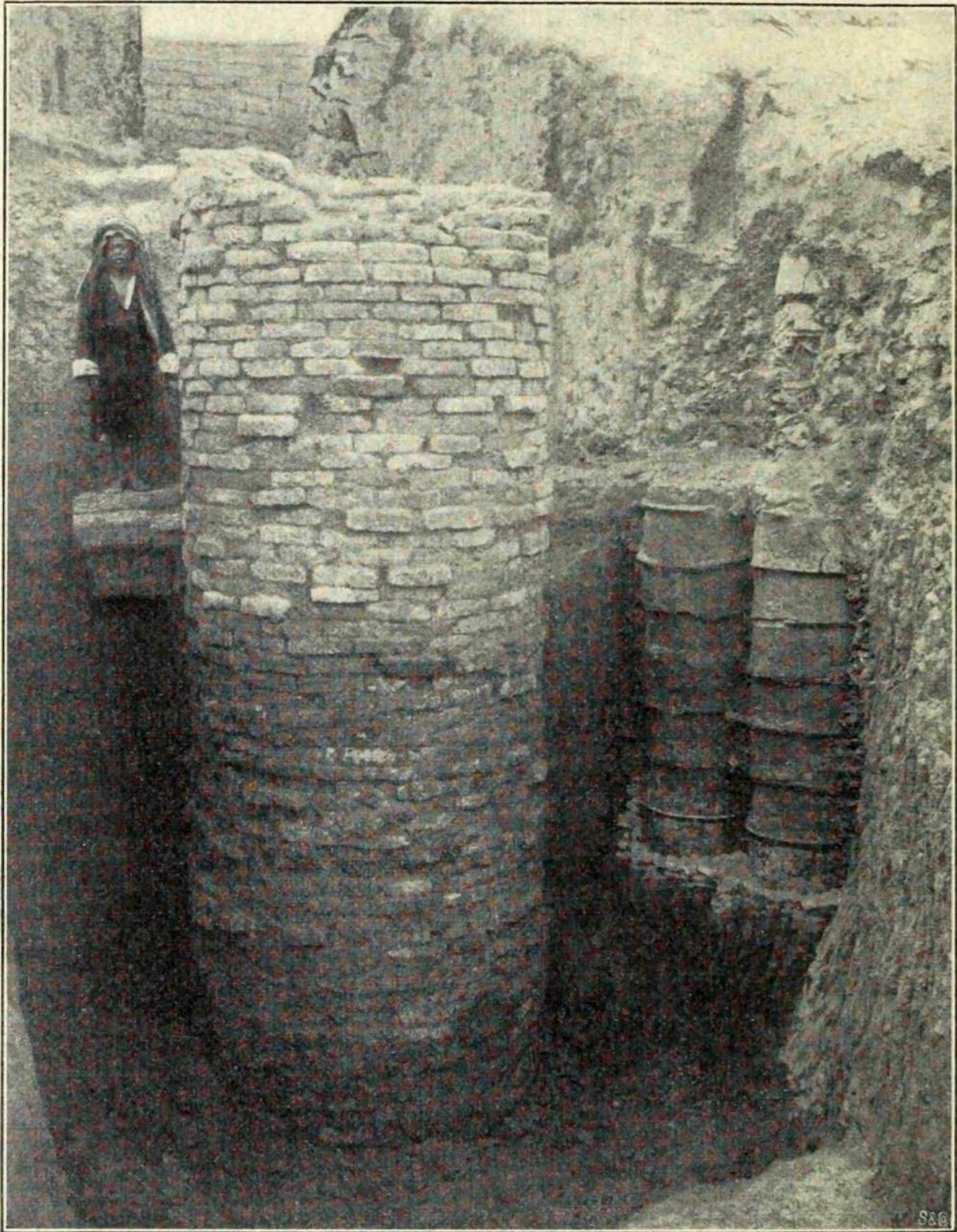
Abb. 24. Grab-Brunnen und Drainierungsröhren aus Terrakotta-Ringen.
