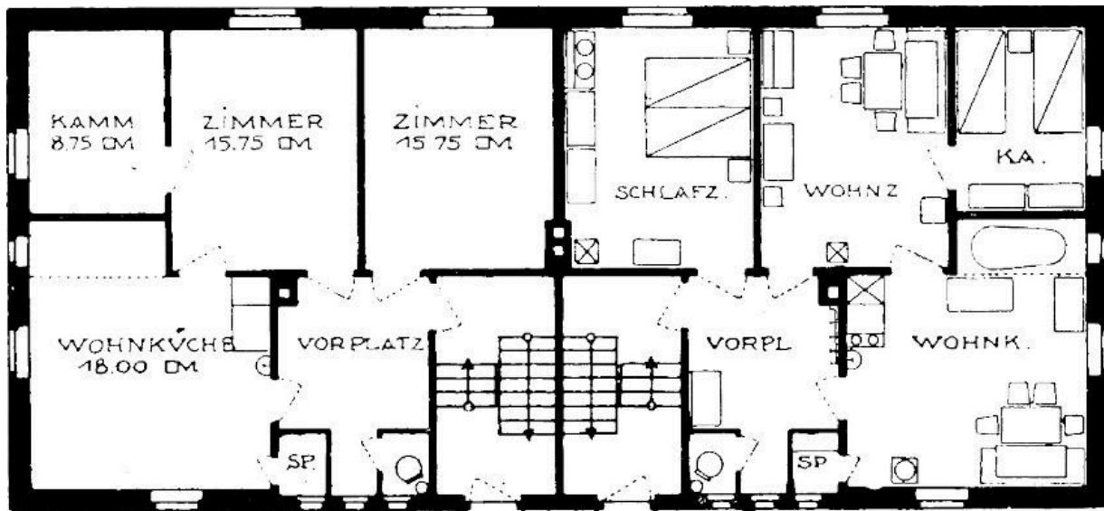
Abb. 4 Doppelwohnhaus für vier Familien der Baumwollspinnerei Zschopau A.-G.
