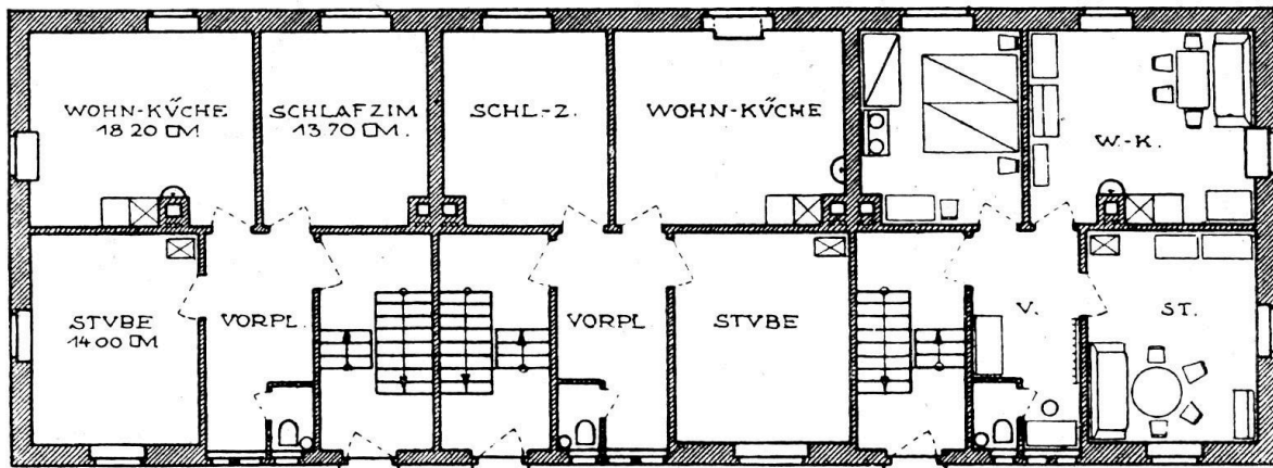
Abb. 3 Doppelwohnhaus für vier Familien der Baumwollspinnerei Zschopau A.-G.
