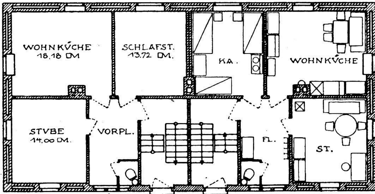
Abb. 7 Gruppenwohnhaus für neun Familien der Baumwollspinnerei Gückelsberg Baukosten 510 909 M.
