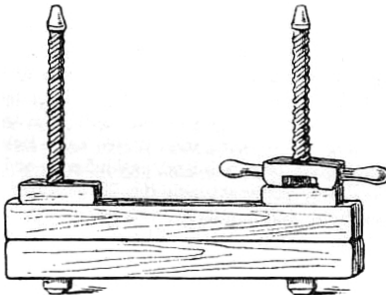
Fig. 4. Handpresse mit Pressbengel.
