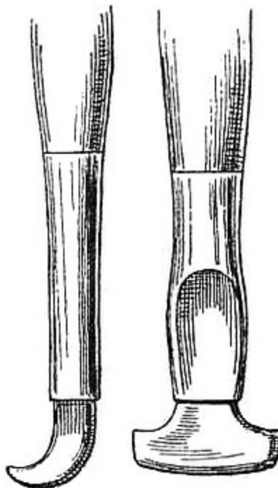
Fig. 39. Glättzähne, flach und rund.
