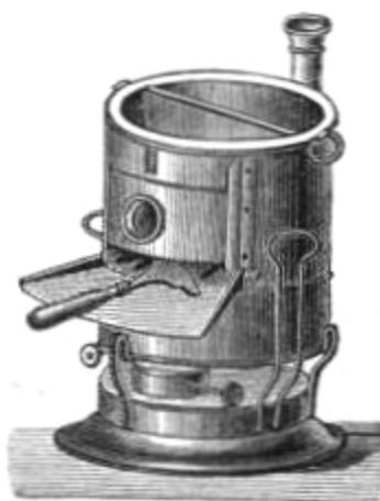
Fig. 26. Leimkessel mit Petroleumheizung von Wilhelm Leo in Stuttgart.
