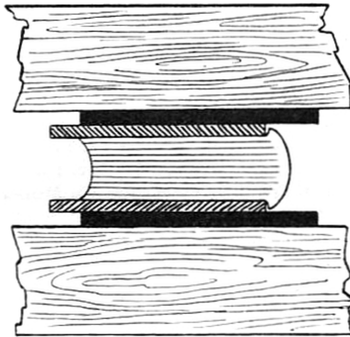
Fig. 41. Zum Vergolden eingesetzter Oberschnitt.
