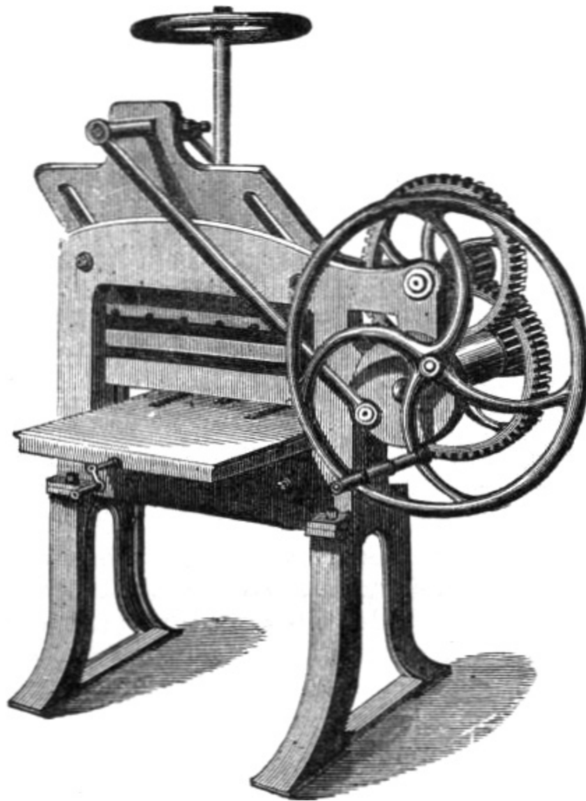
Fig. 24. Beschneidemaschine mit Schwungrad von Dietz & Listing in Leipzig.
