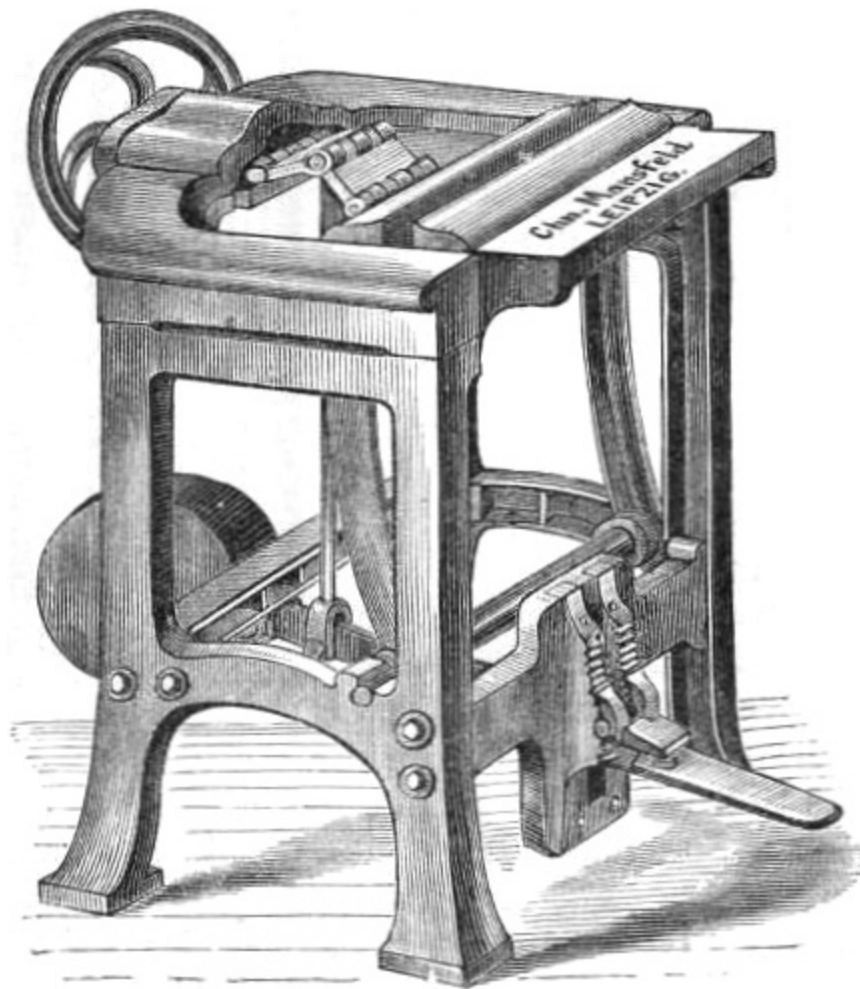
Fig. 20. Abpressmaschine von Chr. Mansfeld in Leipzig.
