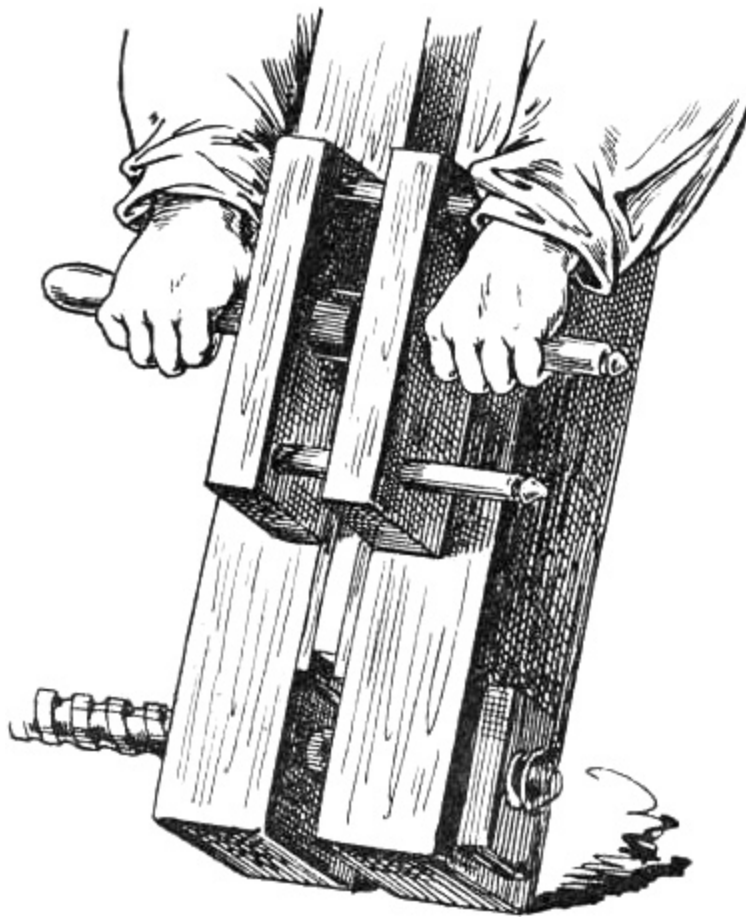
Fig. 21. Beschneiden des Buches.
