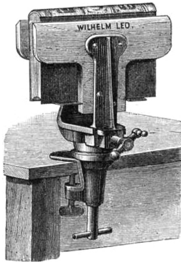
Fig. 66. Klemmvorrichtung von Wilh. Leo in Stuttgart.
