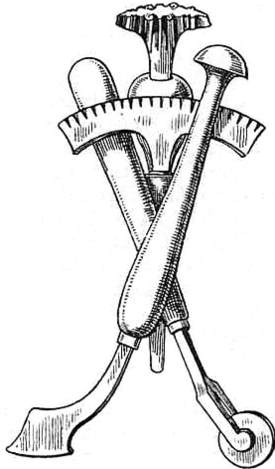
Fig. 64. Streicheisen, Rolle, Stempel und Filet.
