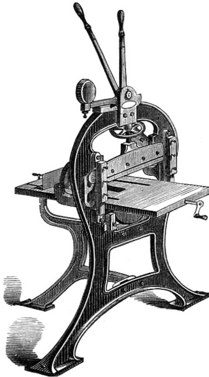
Fig. 23. Beschneidemaschine mit Hebelwerk von Dietz & Listing in Leipzig.
