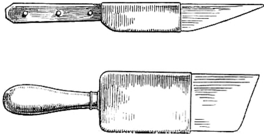
Fig. 53. Offenbacher und Pariser Messerform.
