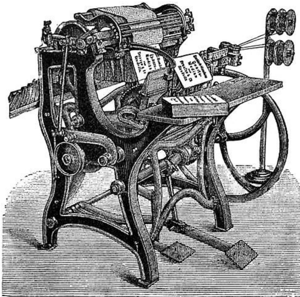
Fig. 13. Drahtheftmaschine von Preuß & Co. in Leipzig.
