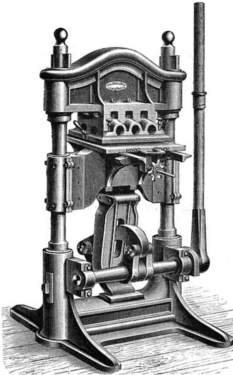
Fig. 105. Vergoldepresse von Mansfeld in Leipzig.
