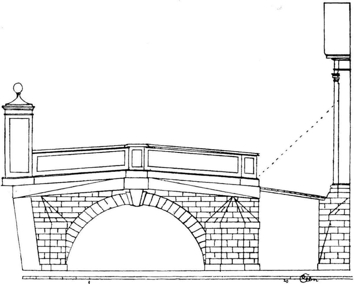
Abb. 3. Der Zwickauer Entwurf für die Frauentorbrücke
