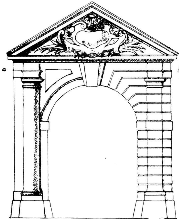
Abb. 2. Naumanns Entwurf für das Portal an der Frauentorbrücke
