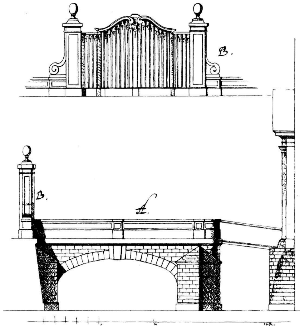
Abb. 4. Pöppelmanns Abänderungsvorschlag zum Zwickauer Entwurf für die Frauentorbrücke (1726)
