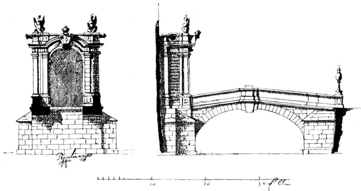
Abb. 1. Pöppelmanns Entwurf für die Niedertorbrücke (1719)
