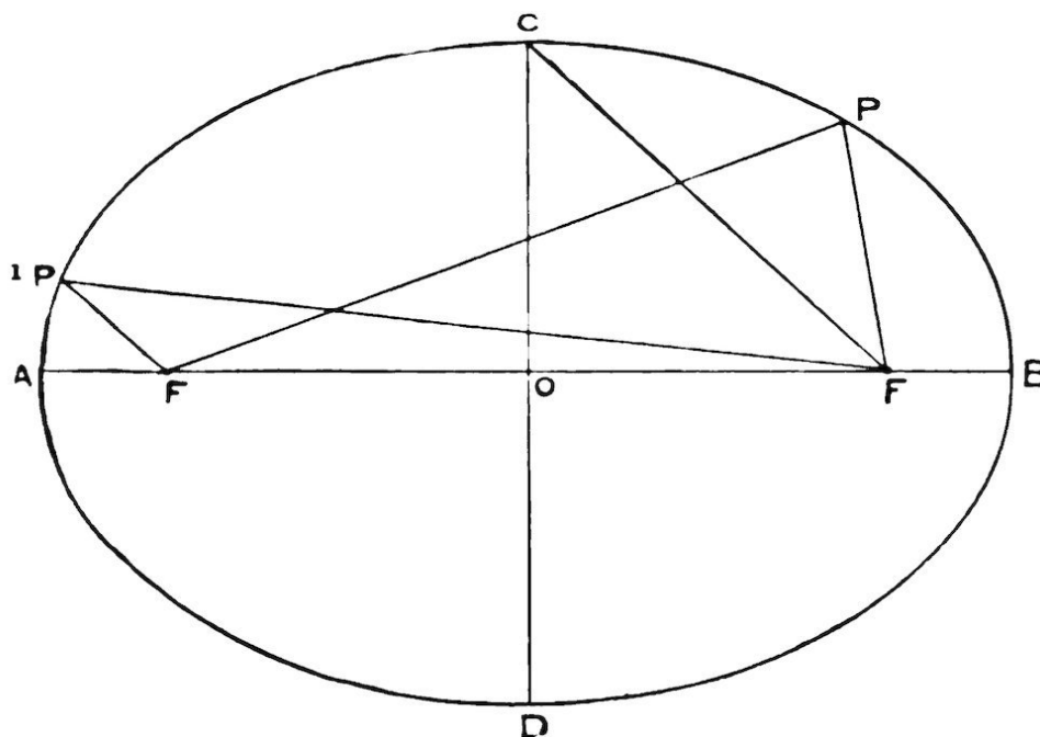
FIG. 14.— The Ellipse.
