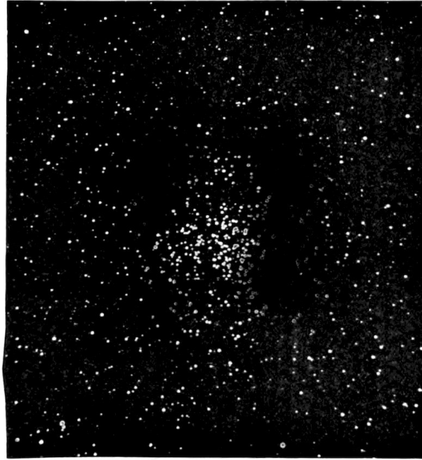
FIG. 11.—37 Messier .
