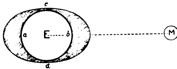
FIG. 45.— The Tides.
