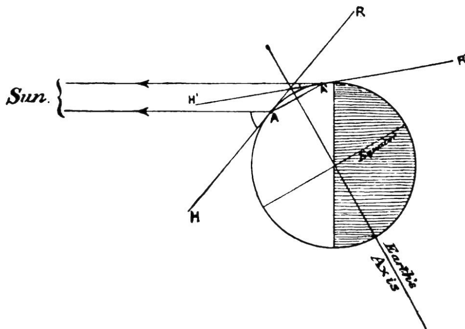
FIG. 10.— The Midnight Sun.
