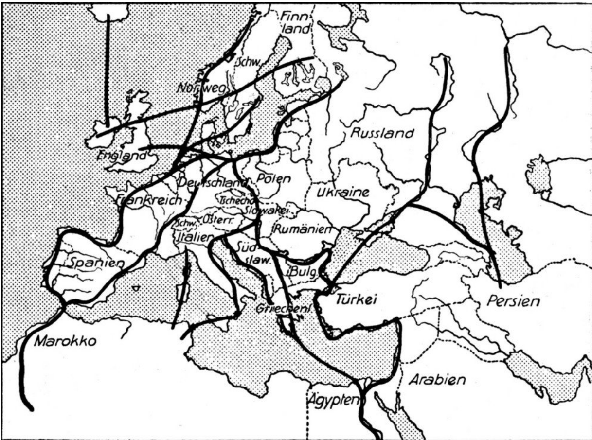
Wichtigste europäische Vogelzugstraßen
