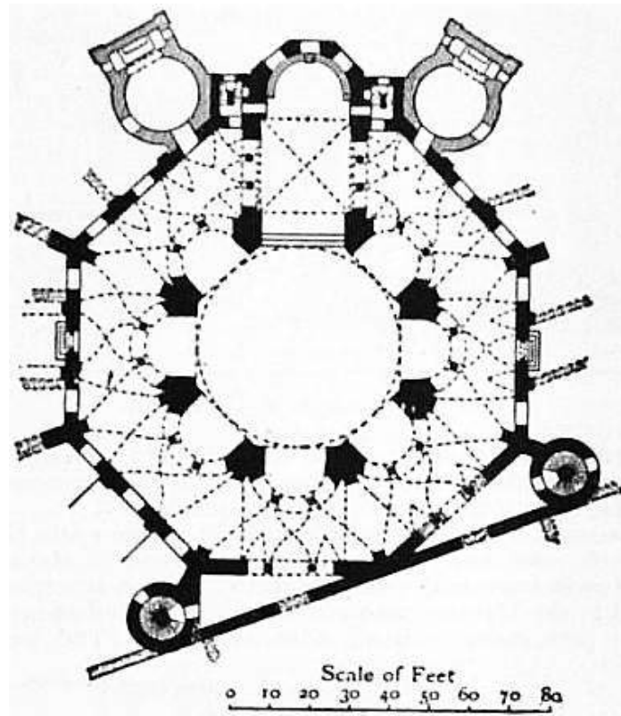
FIG. 30.—Plan of S. Vitale, Ravenna.
