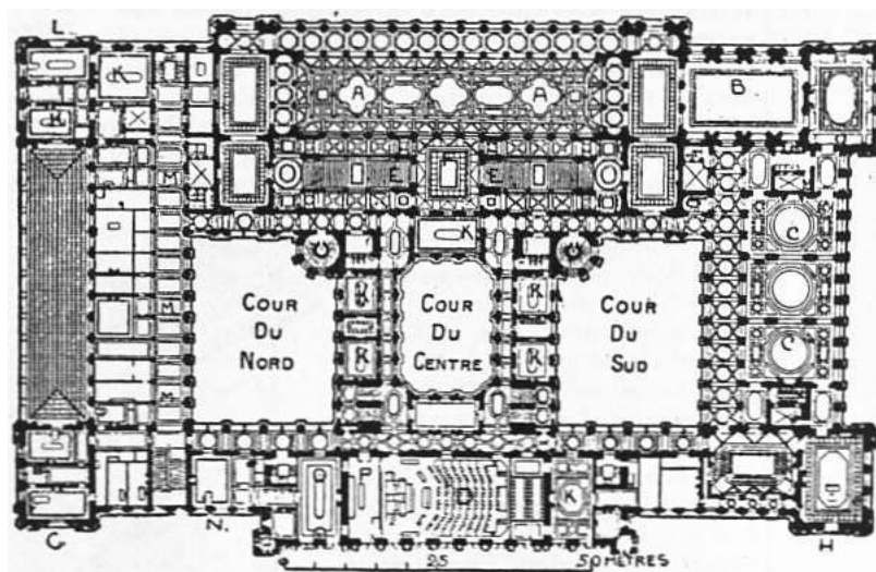
FIG. 109.—Plan of Hôtel de Ville, Paris.
