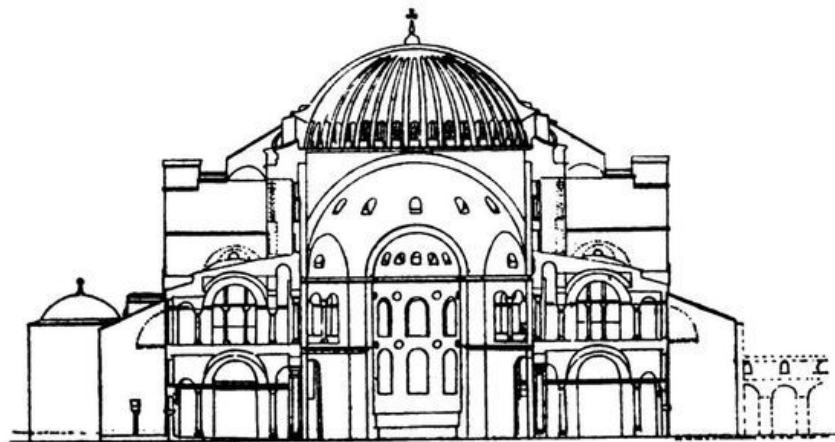
Sainte-Sophie: coupe transversale.
