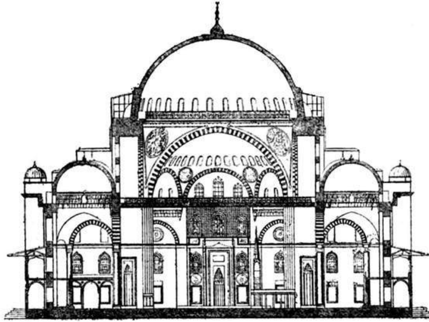
Mosquée Suléïmanié; coupe.
