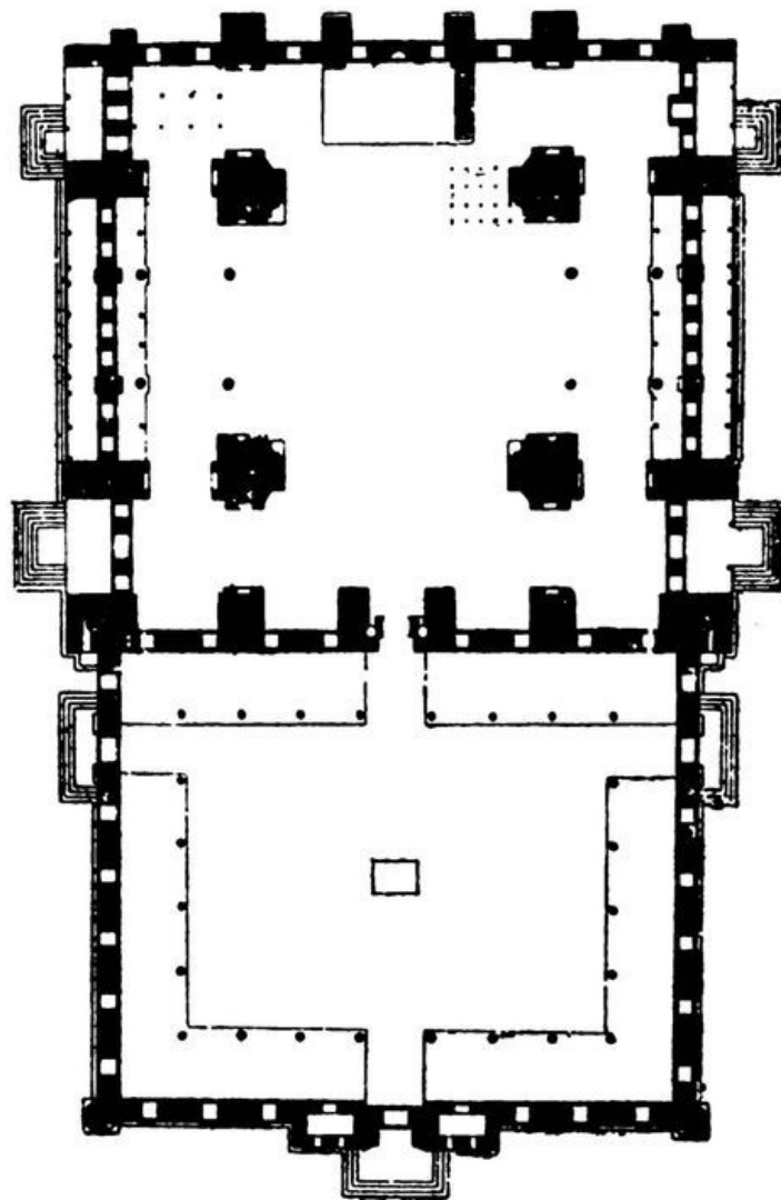
Plan de la mosquée Suléïmanié.
