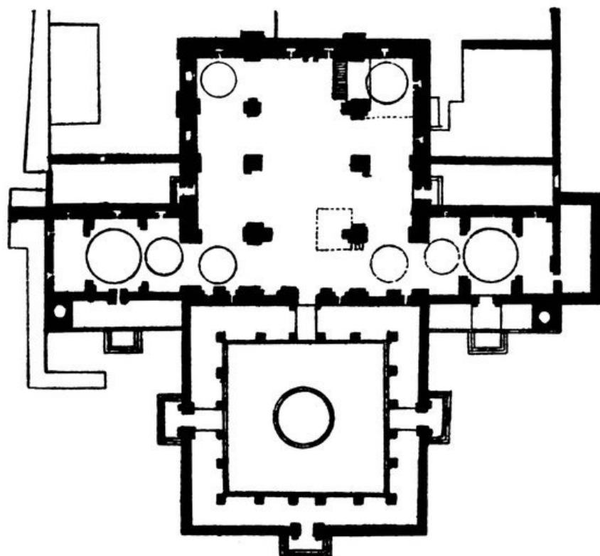
Plan de la mosquée de Bayazid.
