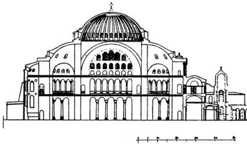
Sainte-Sophie: coupe longitudinale.
