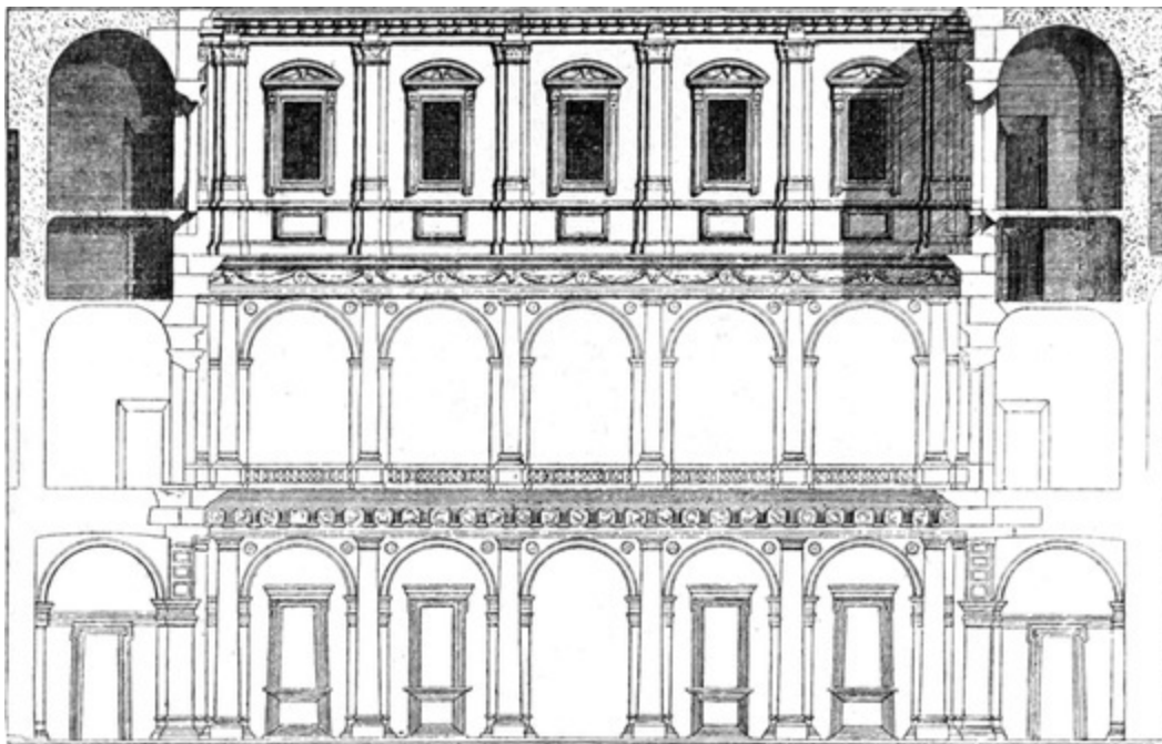
Abb. 74. Hofseite des Palazzo Farnese in Rom (der von Michelangelo entworfene Teil ist durch Schattierung hervorgehoben).
