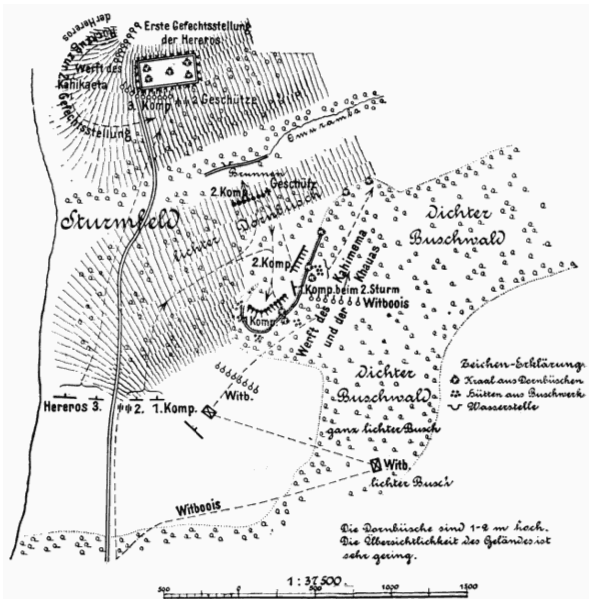
Plan zum Gefecht bei Otjunda-Sturmfeld am 6. Mai 1896.
