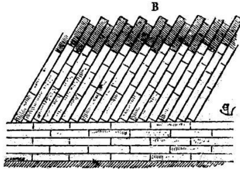
Fig. 2.—Coupe longitudinale.
