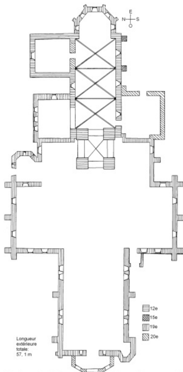
Eglise de Saint-Pair-sur-Mer: plan actuel
