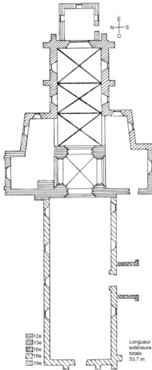
Eglise de Genêts
