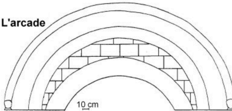
Profil de l'arcade
