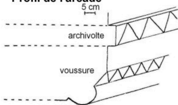
Profil de l'arcade
