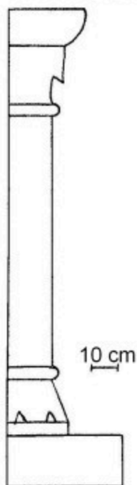
Profil d'une colonne
