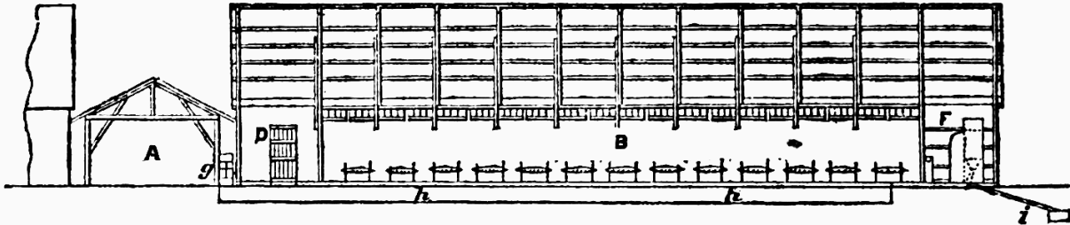
Longitudinal Section.
