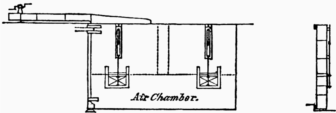
Fig. 21. Brentford Dock Gate.
