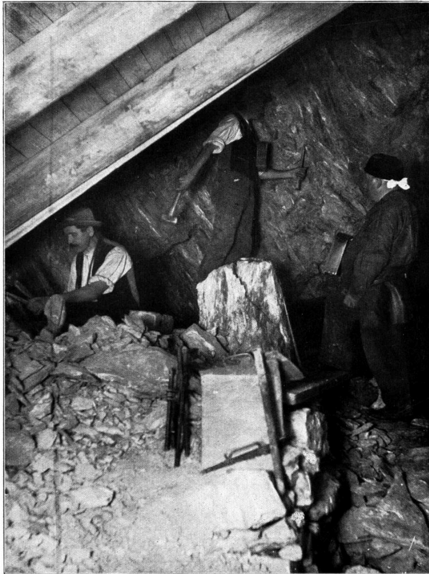
Abb. 18. »Alte Hoffnung Gottes« Kleinvoigtsberg. Streckenstoß in der vierzehnten Gezeugstraße an der Christlich Hilfe Stehenden, sechshundertfünfunddreißig Meter unter Tag.
