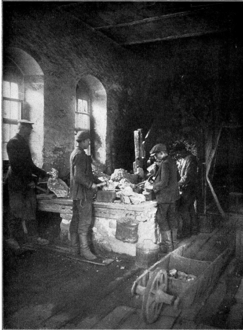
Abb. 13. »Alte Hoffnung Gottes« Kleinvoigtsberg. Scheidebank
