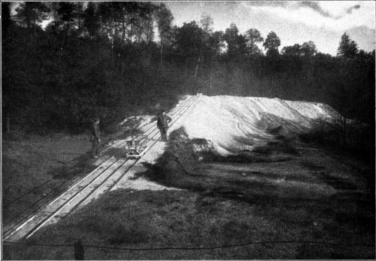
Abb. 17. »Alte Hoffnung Gottes« Kleinvoigtsberg. Aufbereitung, Schlammhalde. Drahtseilbahn mit dressierten Hunten
