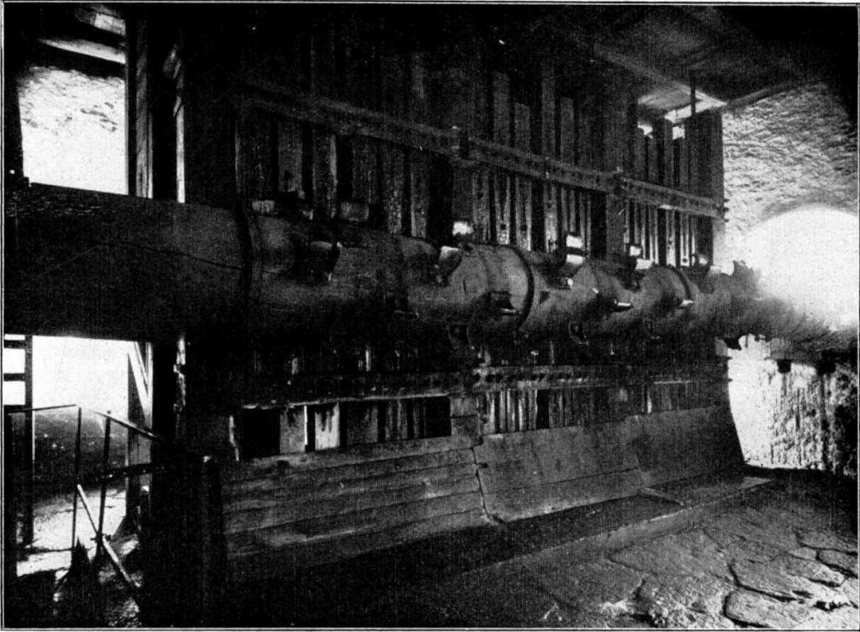
Abb. 14. »Alte Hoffnung Gottes« Kleinvoigtsberg. Naßpochwerk im Niederen Pochhaus
