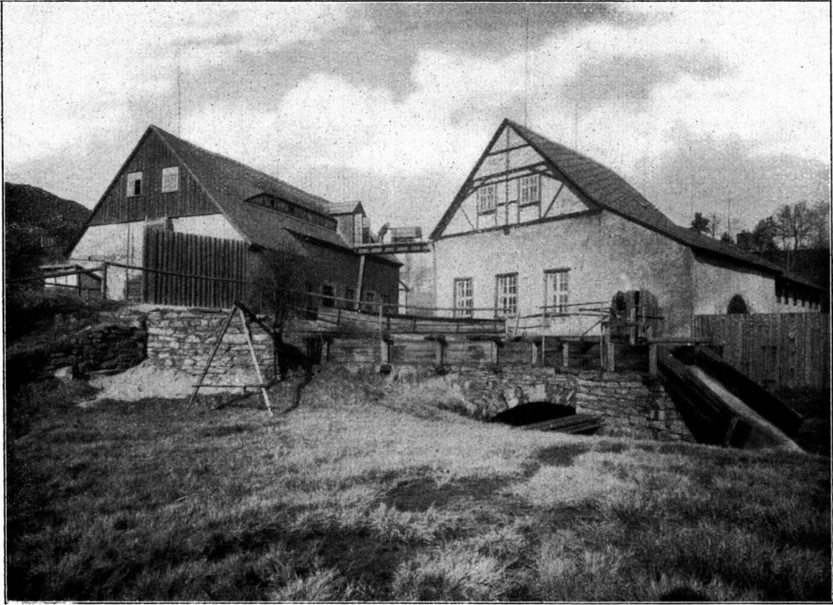
Abb. 12. »Alte Hoffnung Gottes« Kleinvoigtsberg. Oberes und Niederes Pochhaus
