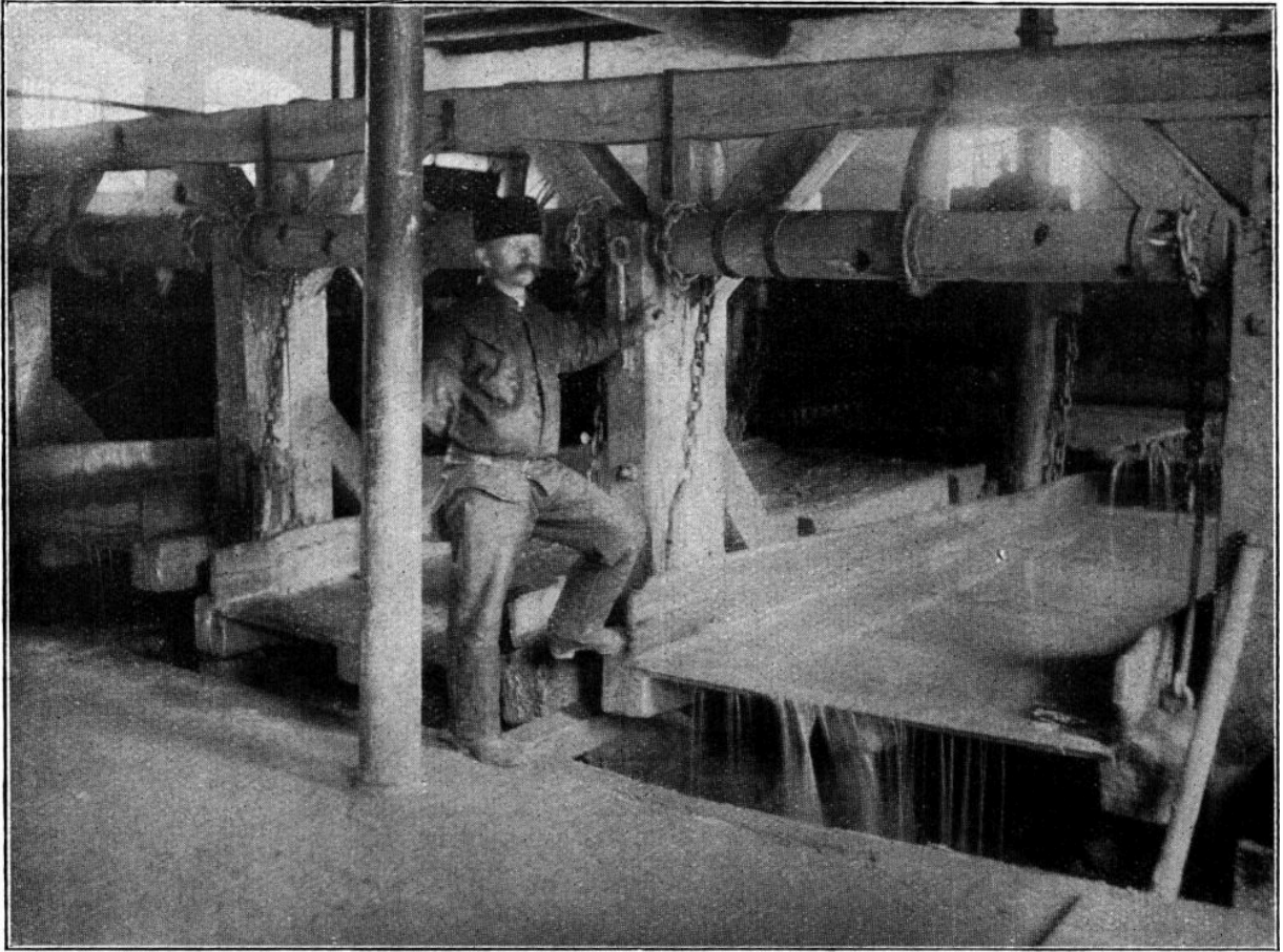
Abb. 16. »Alte Hoffnung Gottes« Kleinvoigtsberg. Aufbereitung, Stoßherde
