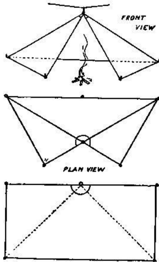
Fig. 2. Rectangle tent
