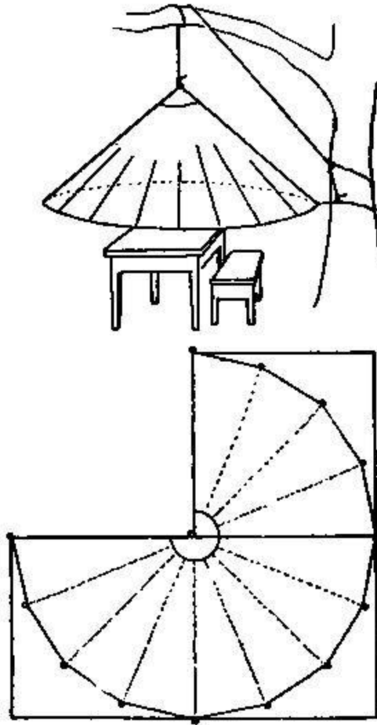
Fig. 11. Sibley awning
