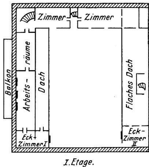
Grundriß eines afghanischen Wohnhauses
