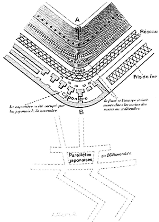
Plan de la caponière du fort de Kekausan-Nord et des parallèles japonaises creusées pour l'attaque.
