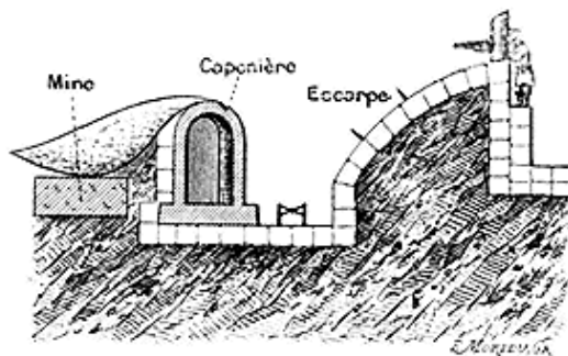
Coupe en A-B de l'escarpe, du fossé et de la caponière du fort de Kekausan-Nord.
