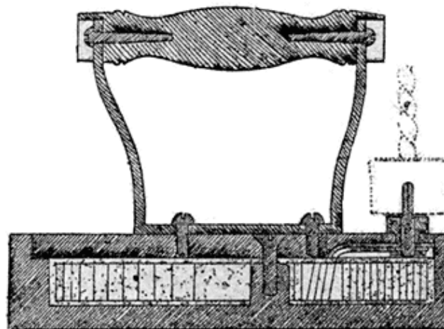
Coupe du fer électrique.
