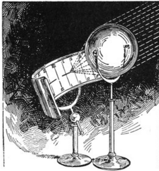
FIG. 3.—A Tell-tale for the Sun.
