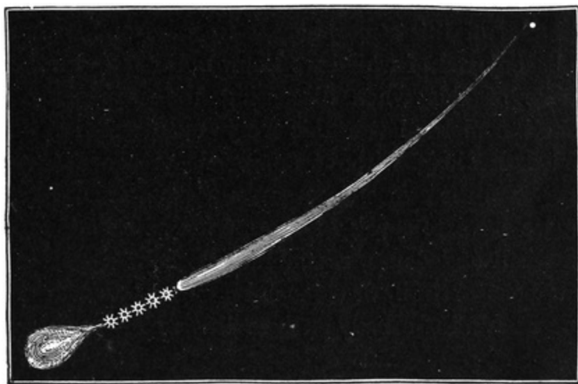
FIG. 77.—A Brilliant Meteor.
