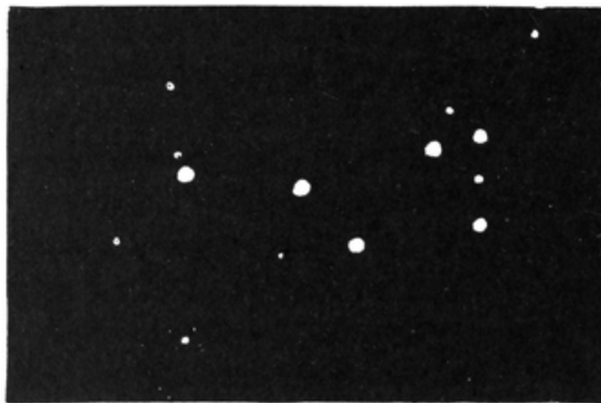
FIG. 89.—The Pleiades.
