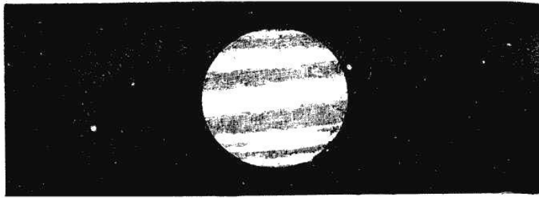
Jupiter
