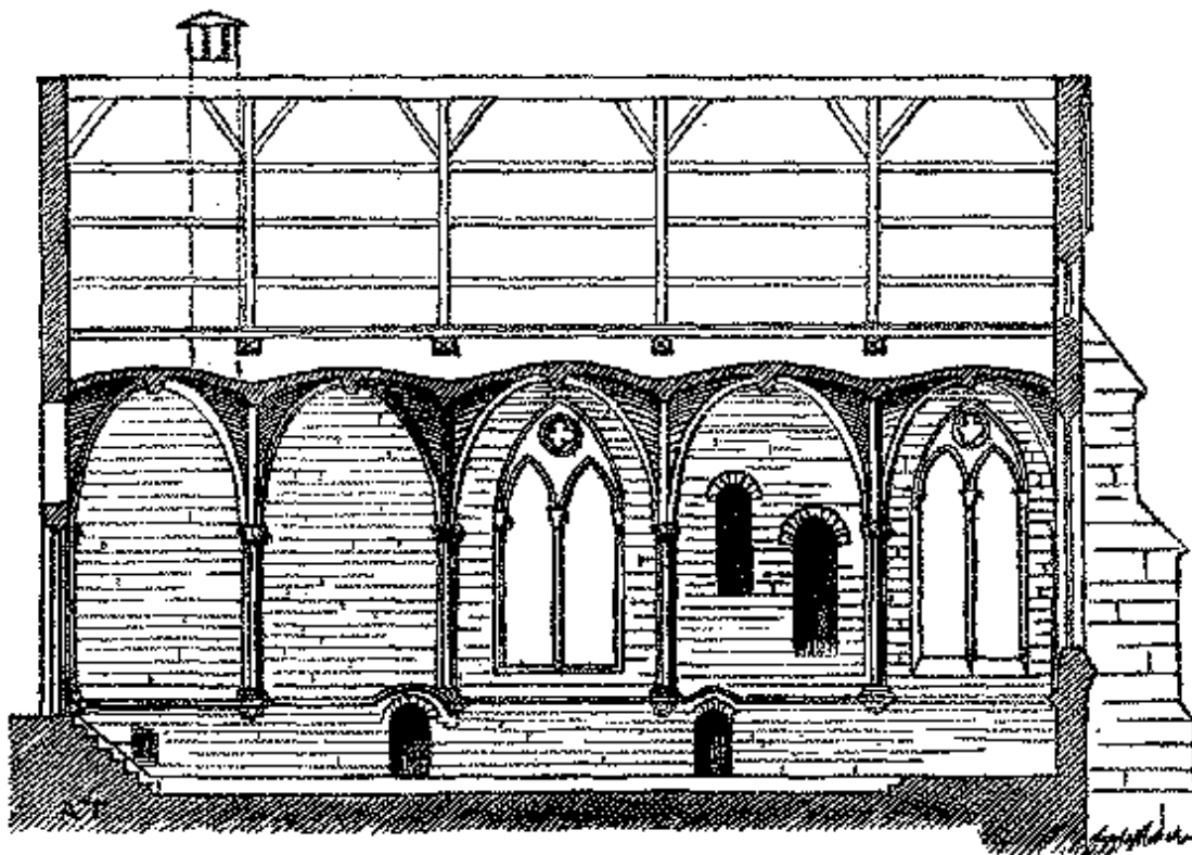
Figura 186: Vista longitudinal do refeitório de Bonport
