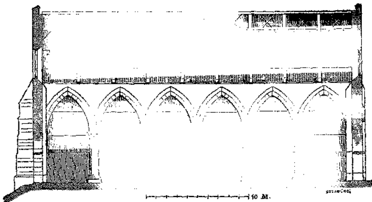
Figura 153: Perfil longitudinal do celleiro de Perrières
