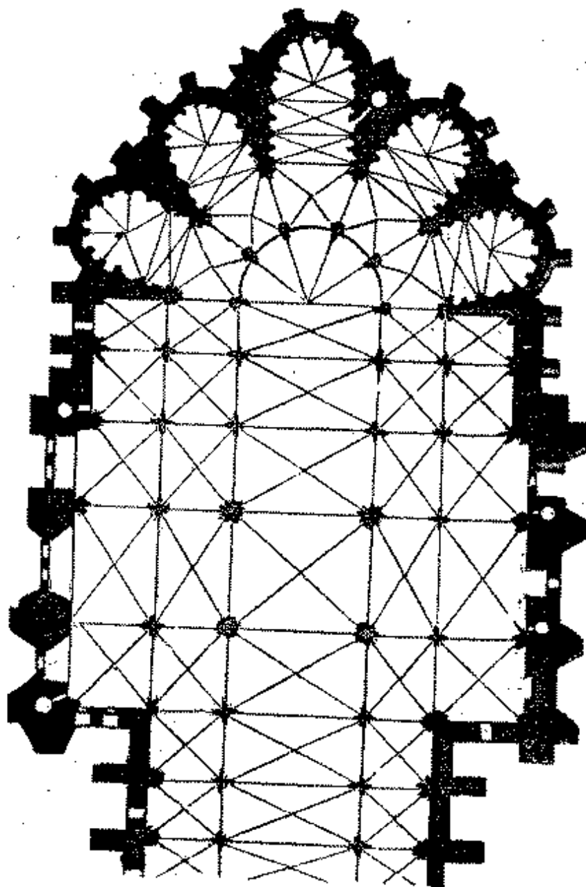
Figura 164: Plano do côro da cathedral de Reims
