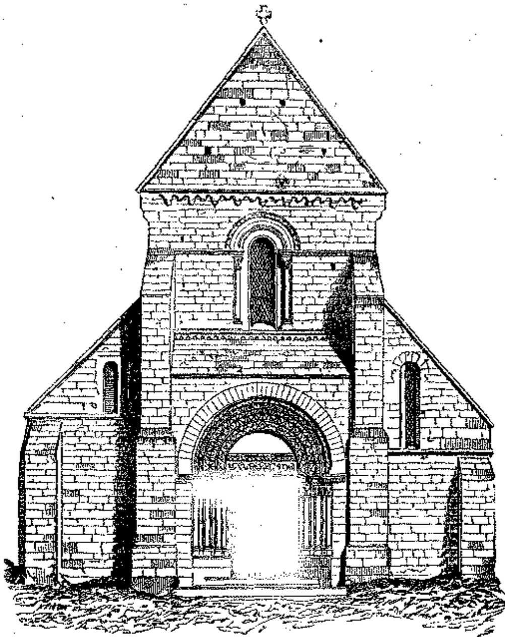
Figura 134: Fachada da igreja de Jort (Calvados).
