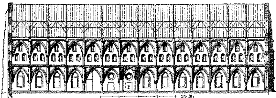
Figura 190: Côte longitudinal d'esse edificio
