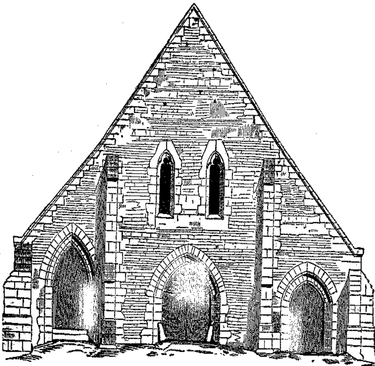
Figura 194: Entrada do mercado de Saint-Pierre-sur-Dive
