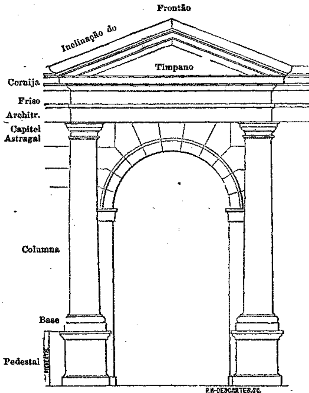
Figura 34: Portico da Ordem Toscana
