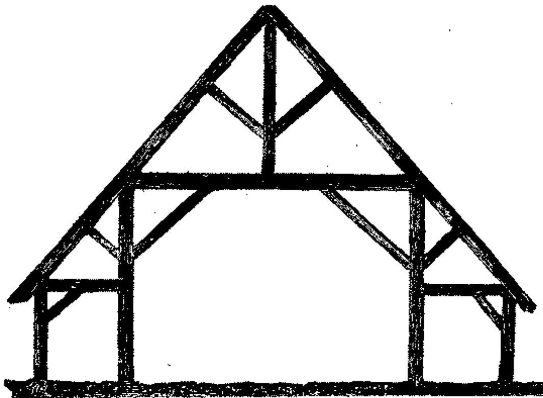
Figura 226: Córte transversal do mercado de Dives
