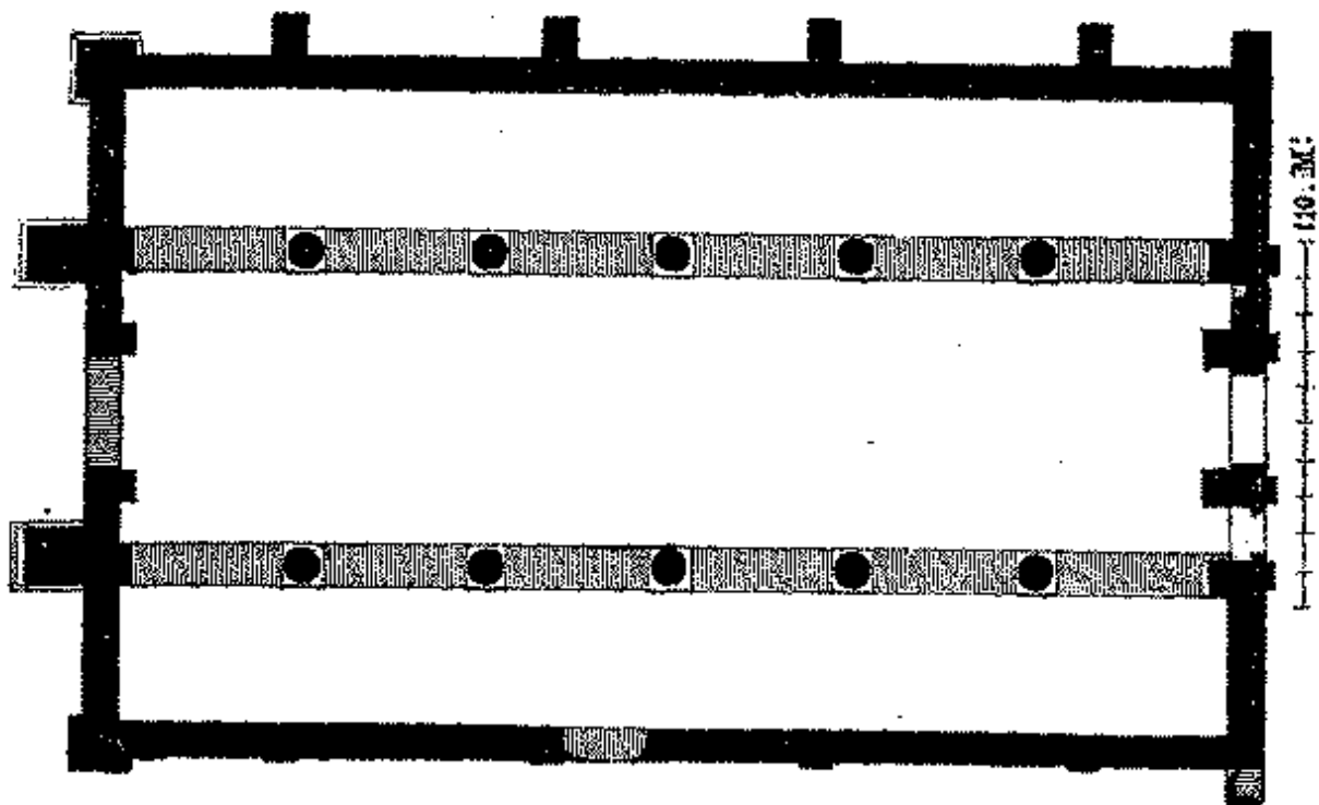
Figura 152: Plano do celleiro de Perrières
