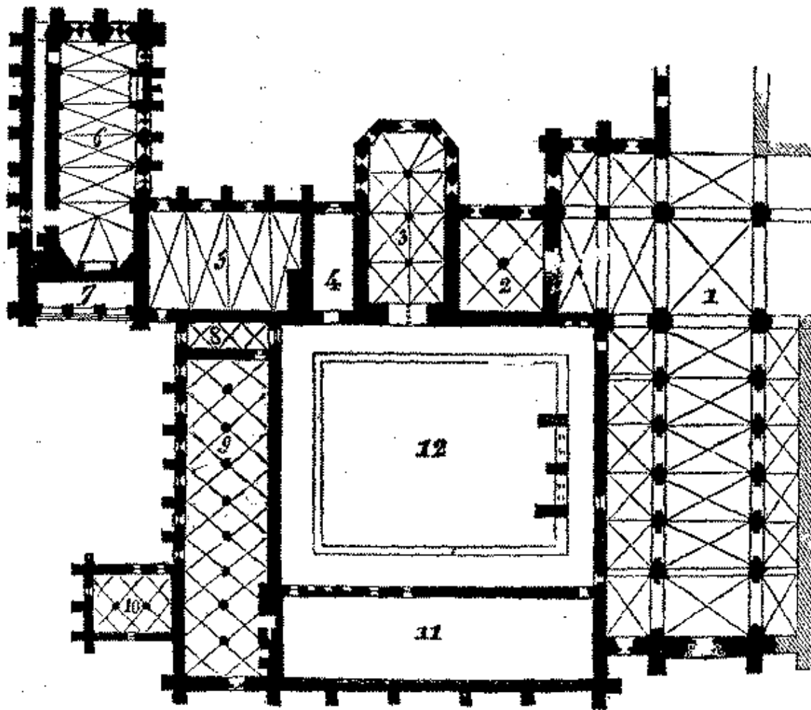
Figura 150: Plano d'uma abbadia do seculo XII (parte central) 1, igreja. 3, sala capítular. 2, 4, 5, salas abobadadas, com os dormitorios em volta. 9, refeitório. 11, salas de recepção. 12, pateo rodeado pela galeria do claustro.
