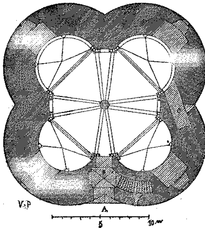
Figura 160: Plano do torreão d'Étampes
