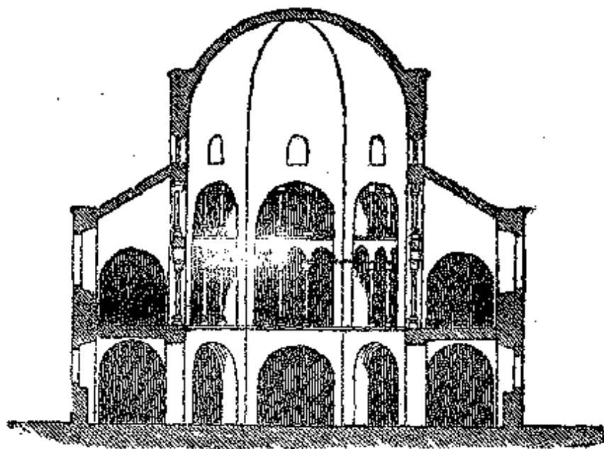
Figura 102: Côte da igreja de Ottmarsheim (Alto Rheno)
