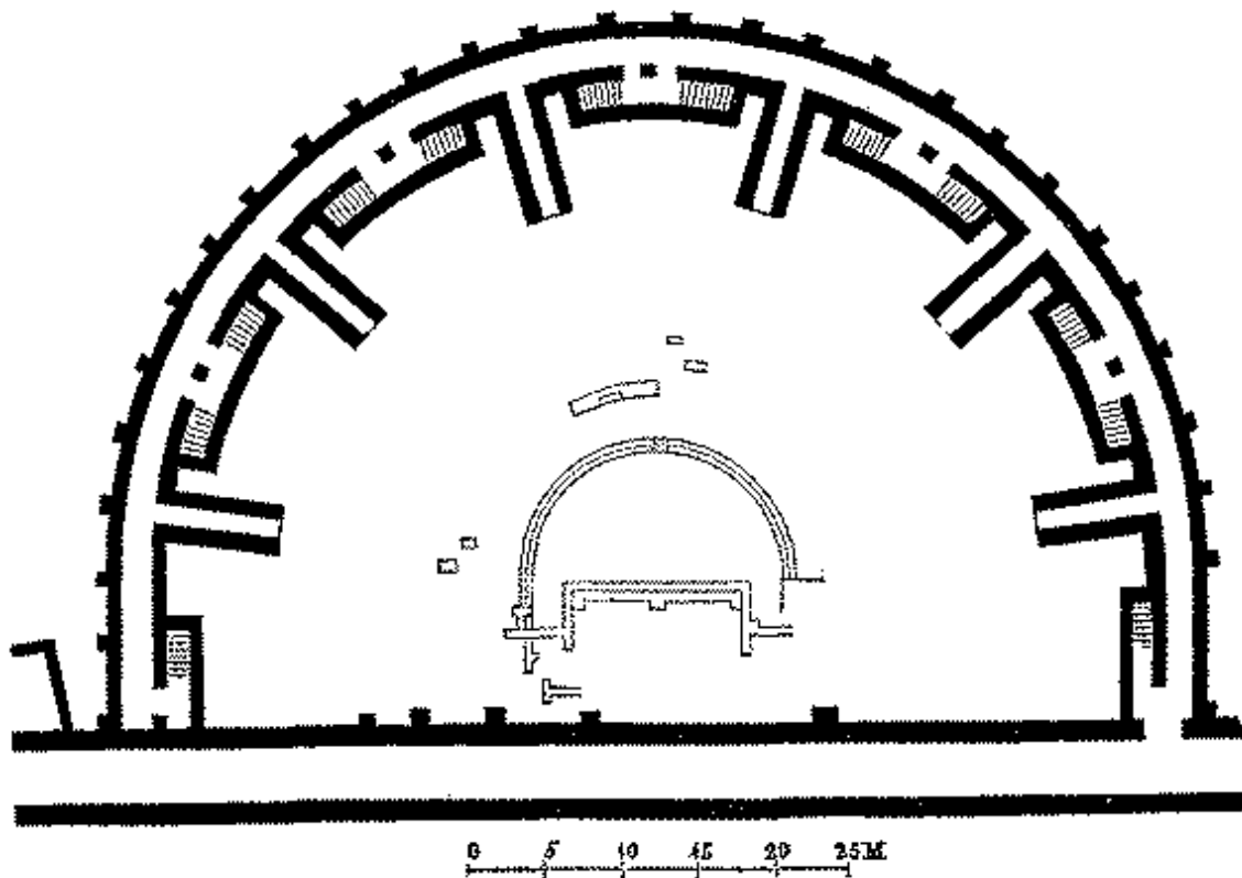
Figura 58: Plano do theatro de Champlieu
