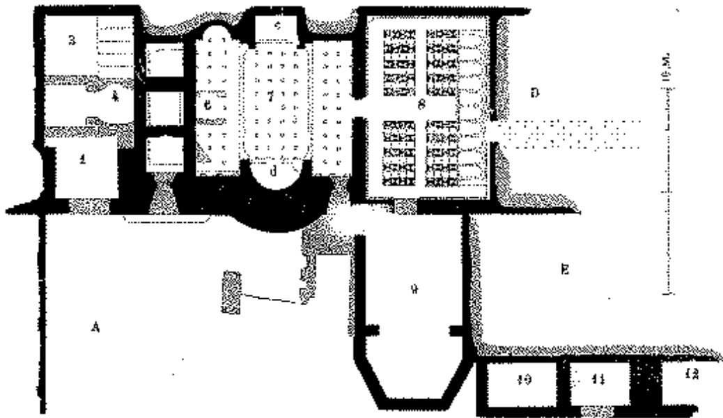
Figura 68: Plano dos banhos de Landunum (França).
