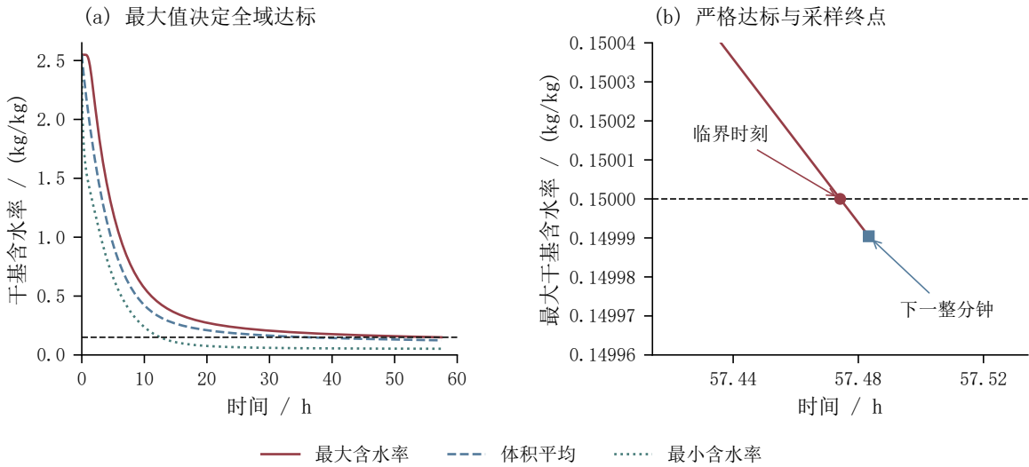
图 11 全域达标与终止时间
