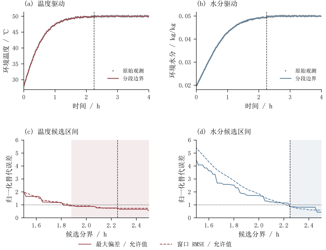
图3 环境边界与分界筛选
