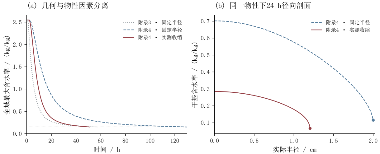
图 19 附录 4 下的收缩对照及与问题 3 的区别
