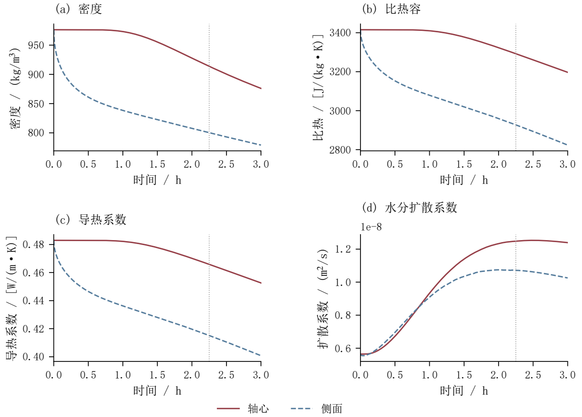
图 7 主要材料参数随时间的动态变化
