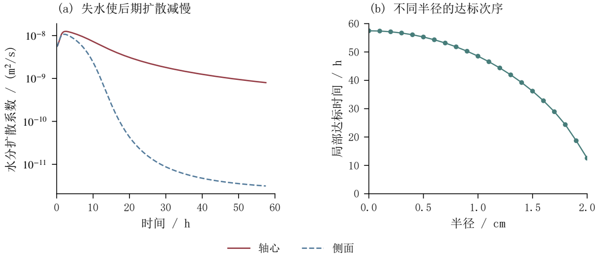
图 13 扩散减慢与局部达标次序
