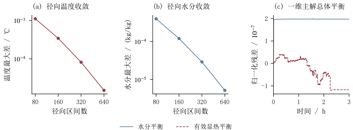
图 8 问题 2 数值收敛性与总体平衡检验
