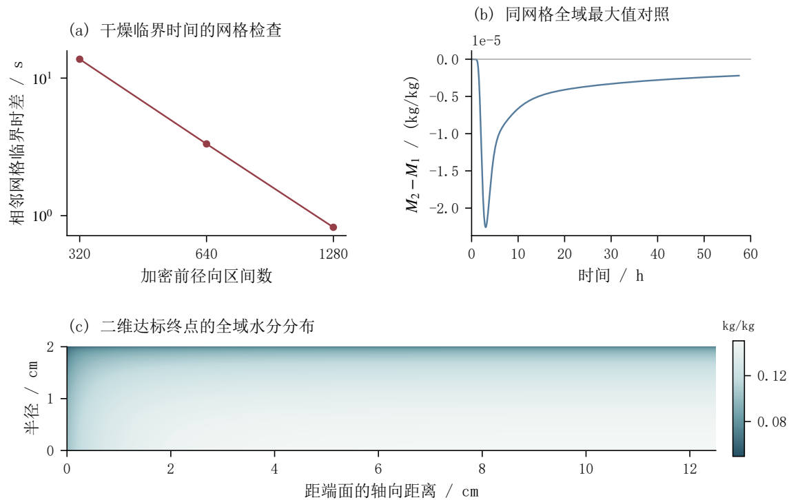
图 14 终止时间的数值与维度检验
