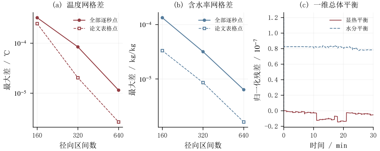
图2 一维网格与总体平衡检验
