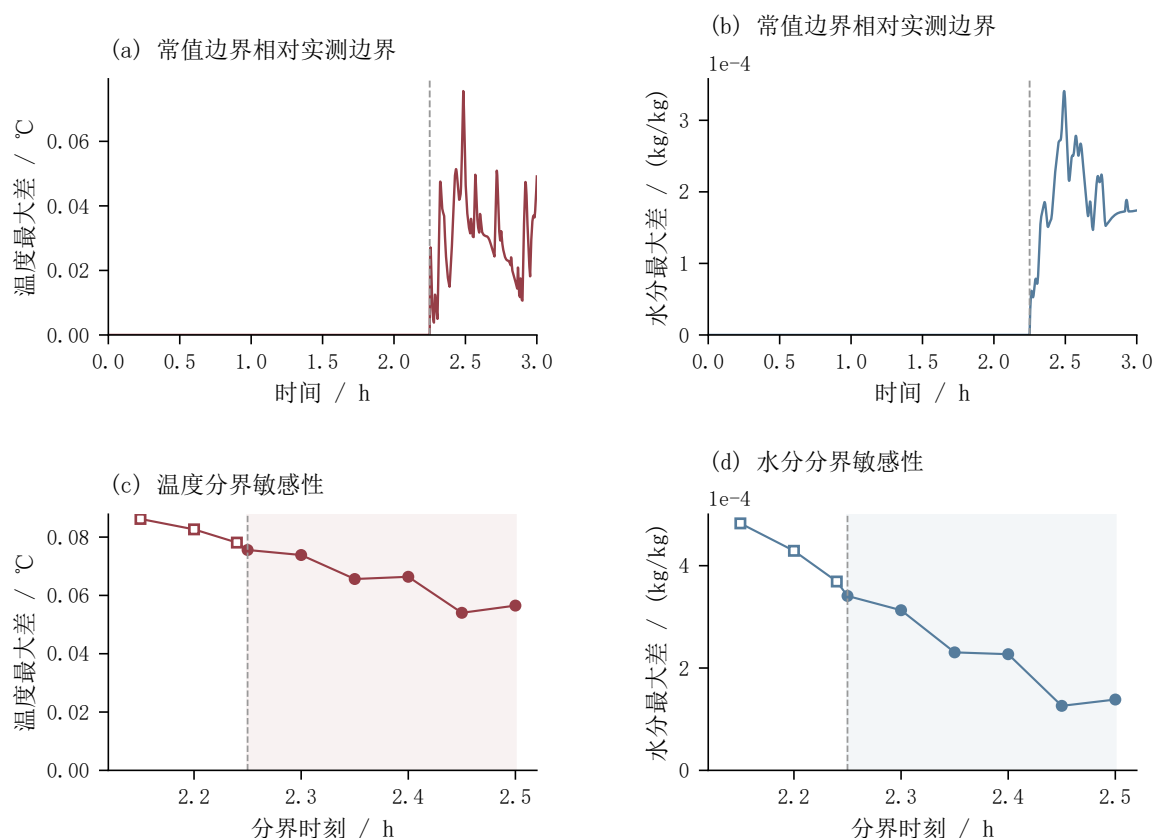
图 10 环境分界的敏感性分析
