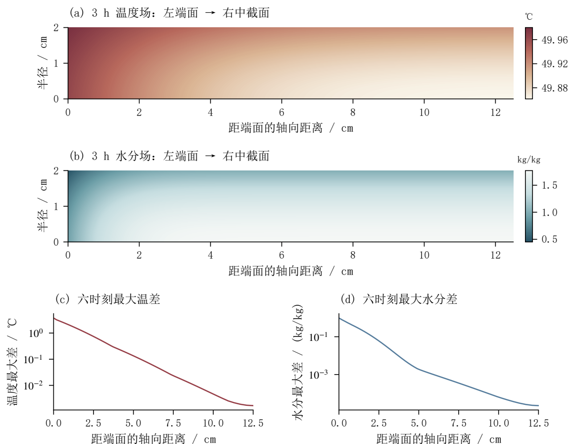
图 9 轴向传递引起的空间差异
