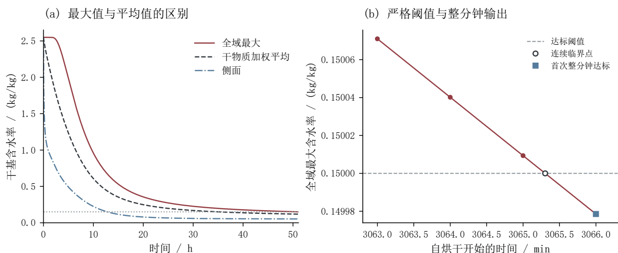
图 22 全域达标判据及终止时刻的局部核验
