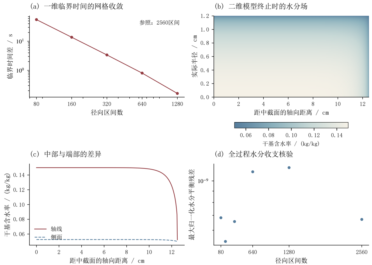
图 24 网格收敛、二维端部差异及水分收支检验
