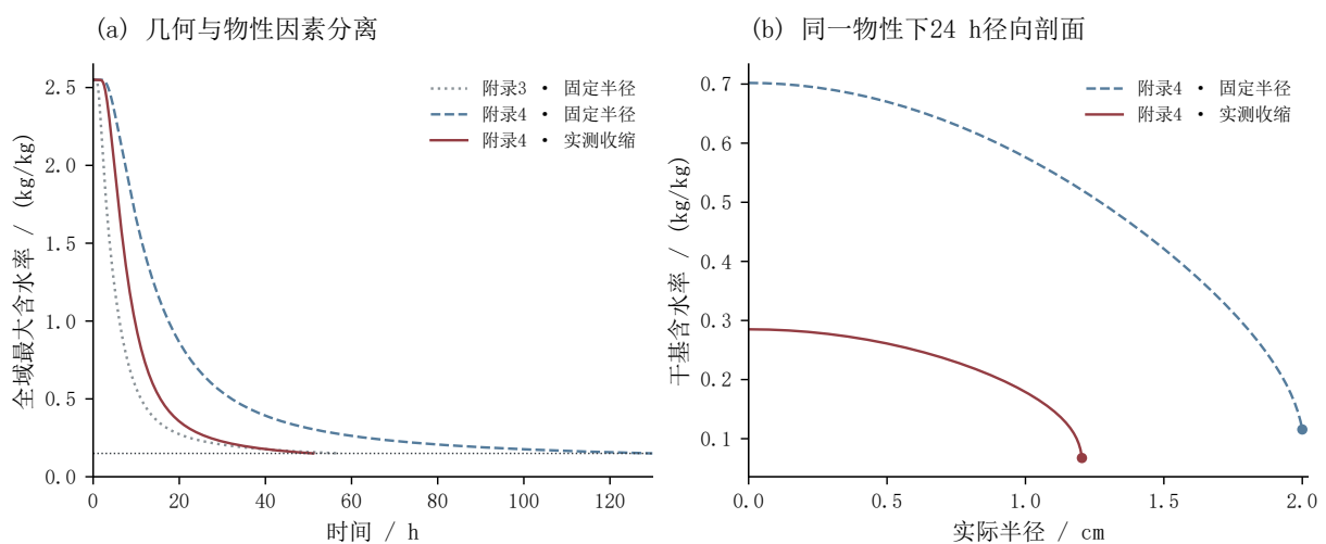
图 23 附录 4 下的收缩对照及与问题 3 的区别
