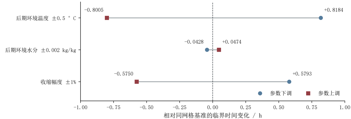
图 25 后期环境与收缩幅度对临界时间的影响
