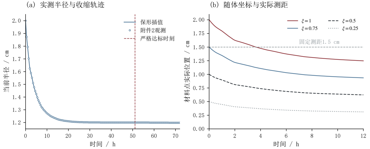
图 20 实测收缩与随体径向坐标
