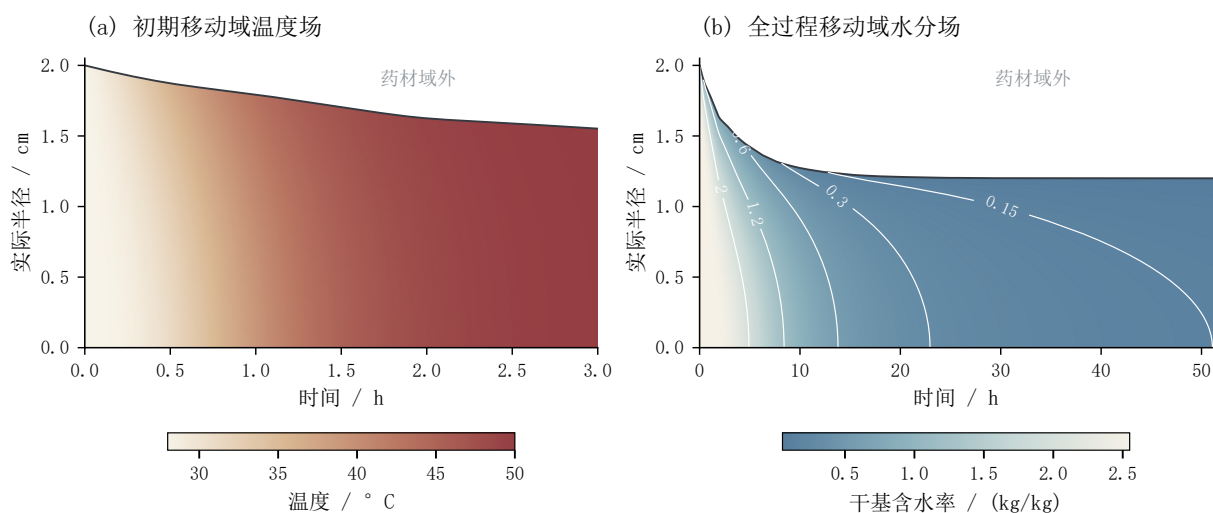
图 21 收缩域内的温度与干基含水率演化
