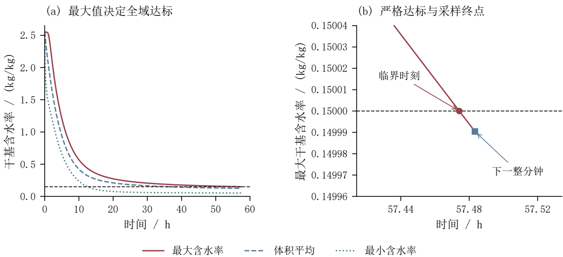
图 15 全域达标与终止时间
