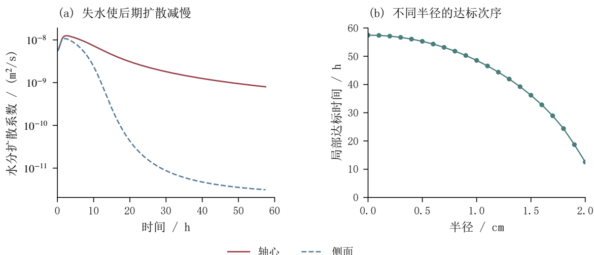
图 17 扩散减慢与局部达标次序
