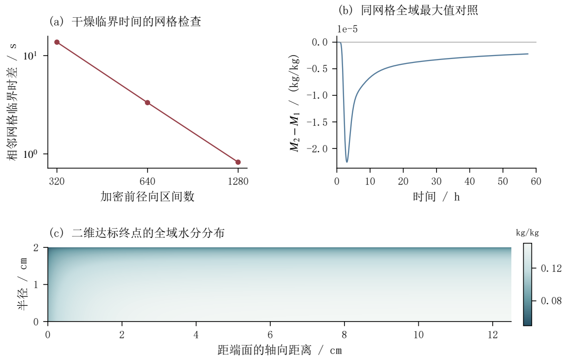
图 18 终止时间的数值与维度检验
