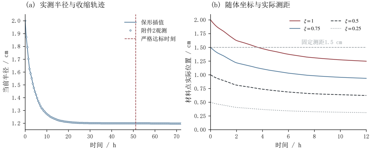
图 18 实测收缩与随体径向坐标
