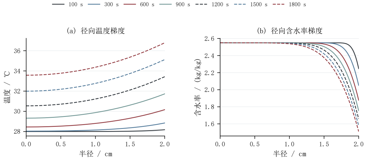
图3 指定时刻的径向状态剖面
