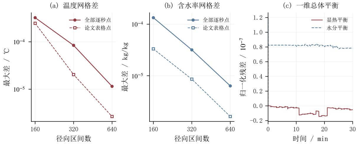
图4 一维网格与总体平衡检验
