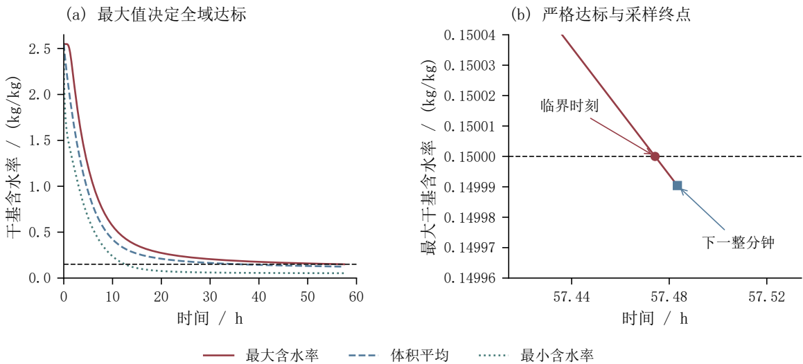
图 13 全域达标与终止时间
