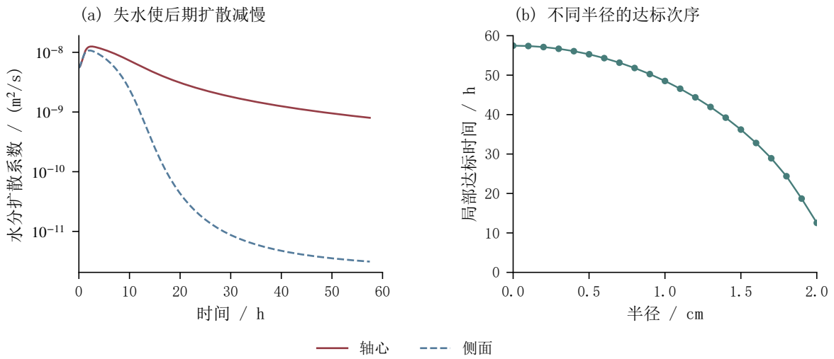
图 15 扩散减慢与局部达标次序
