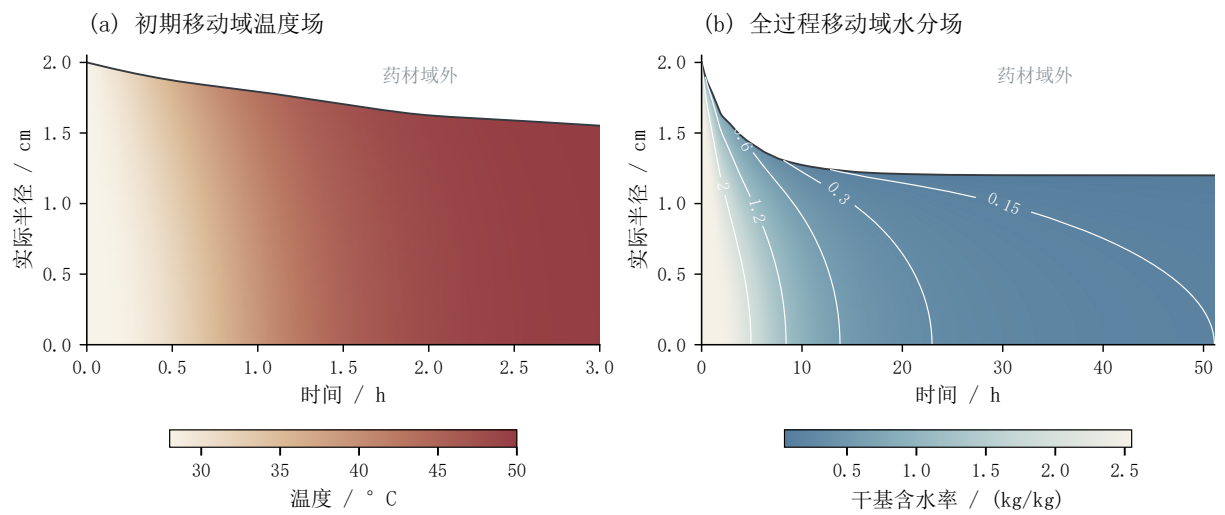
图 19 收缩域内的温度与干基含水率演化
