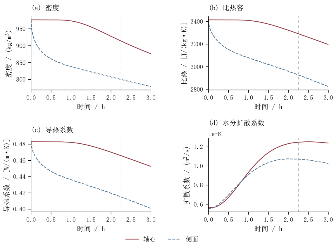
图 9 主要材料参数随时间的动态变化
