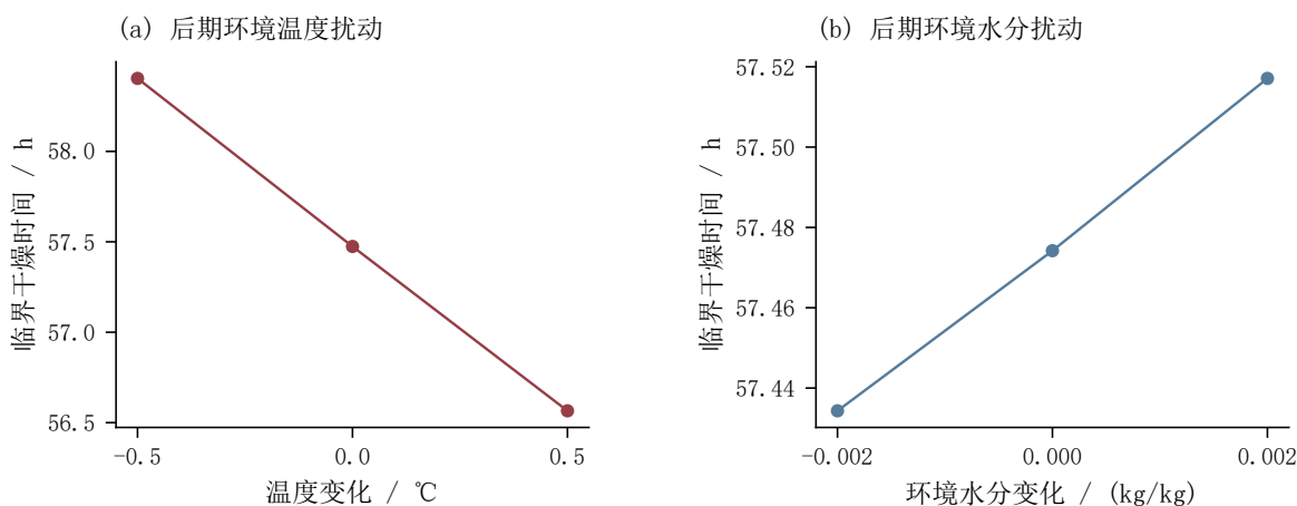
图 17 后期平台对干燥时长的影响
