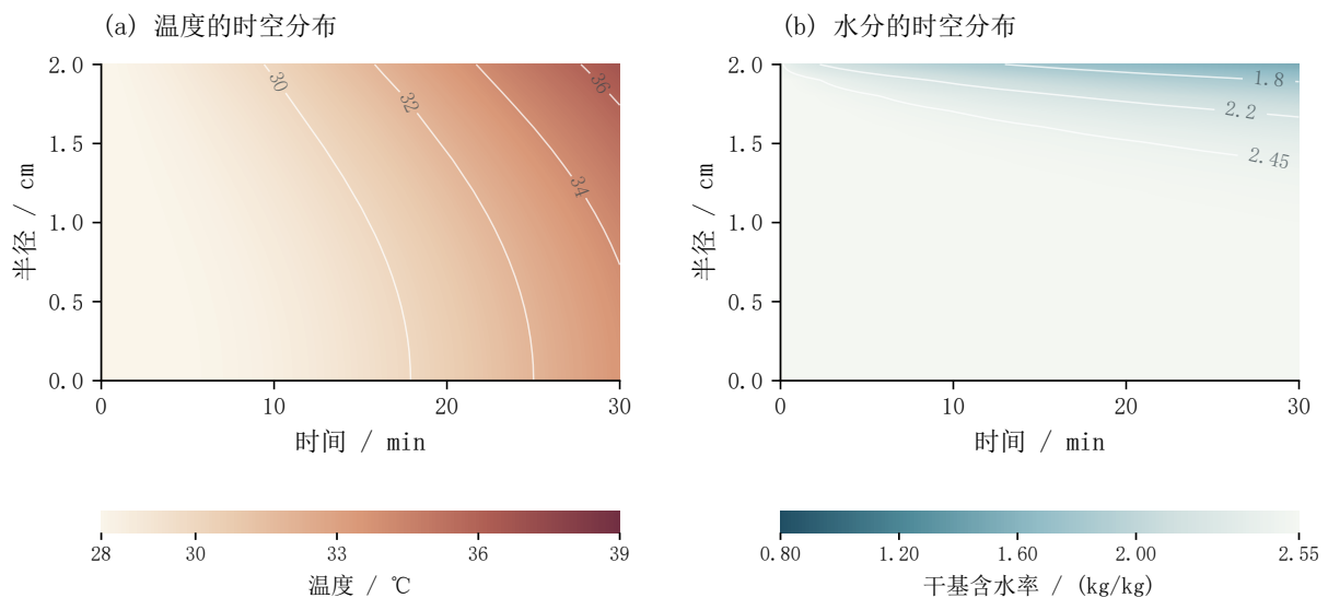
图 2 一维温湿状态的时空演化
