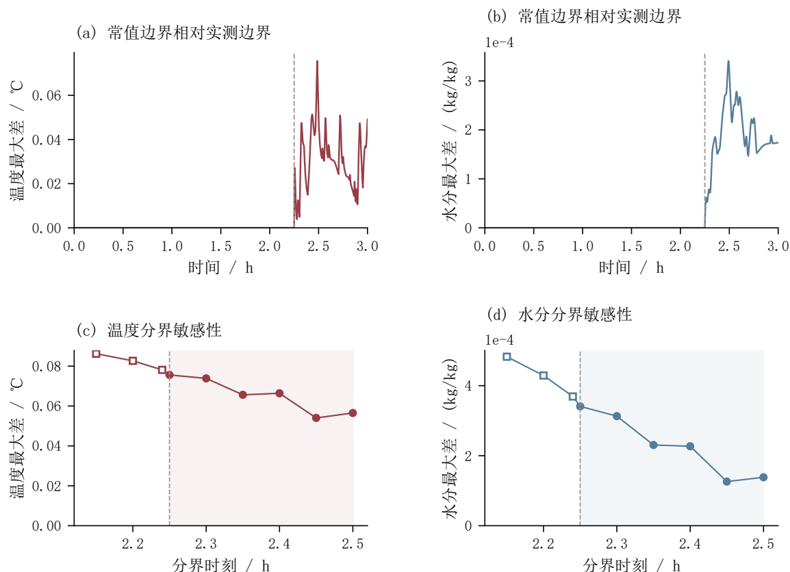
图 12 环境分界的敏感性分析
