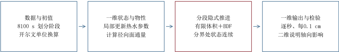
图 6 问题 2 动态参数热湿耦合求解流程
