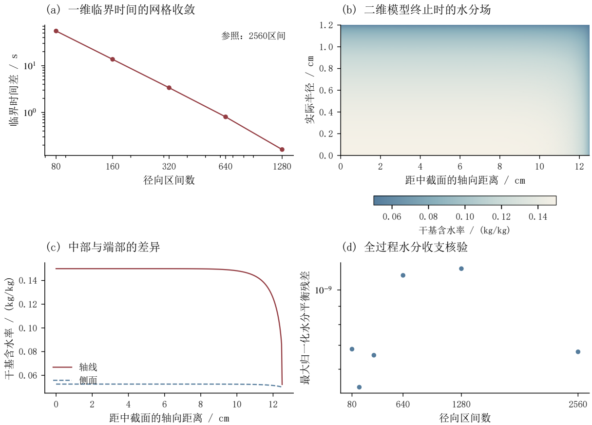
图 22 网格收敛、二维端部差异及水分收支检验
