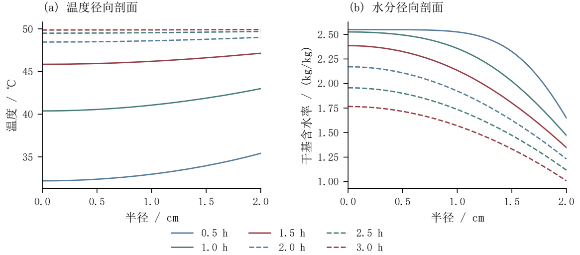
图5 六个规定时刻的径向分布
