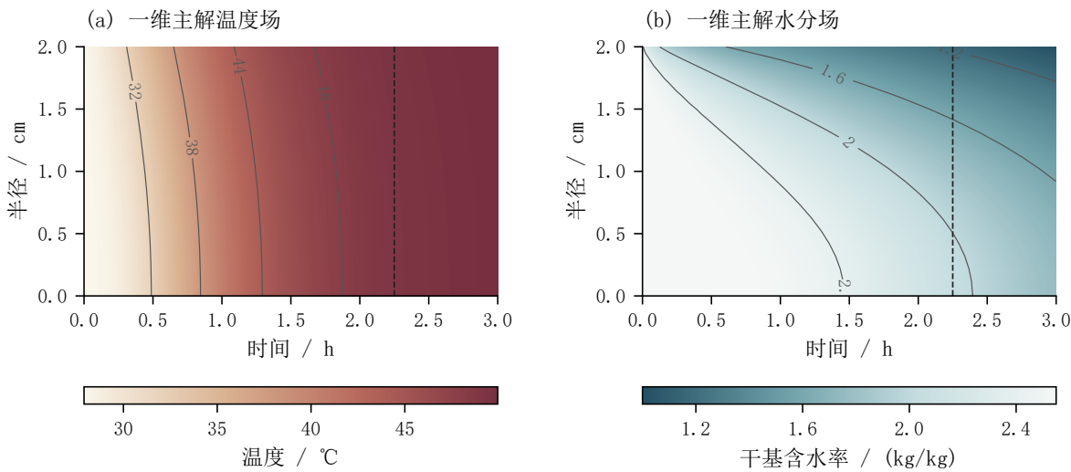
图 4 一维模型温度与含水率的时空分布
