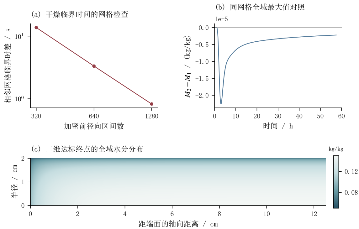
图 18 终止时间的数值与维度检验
