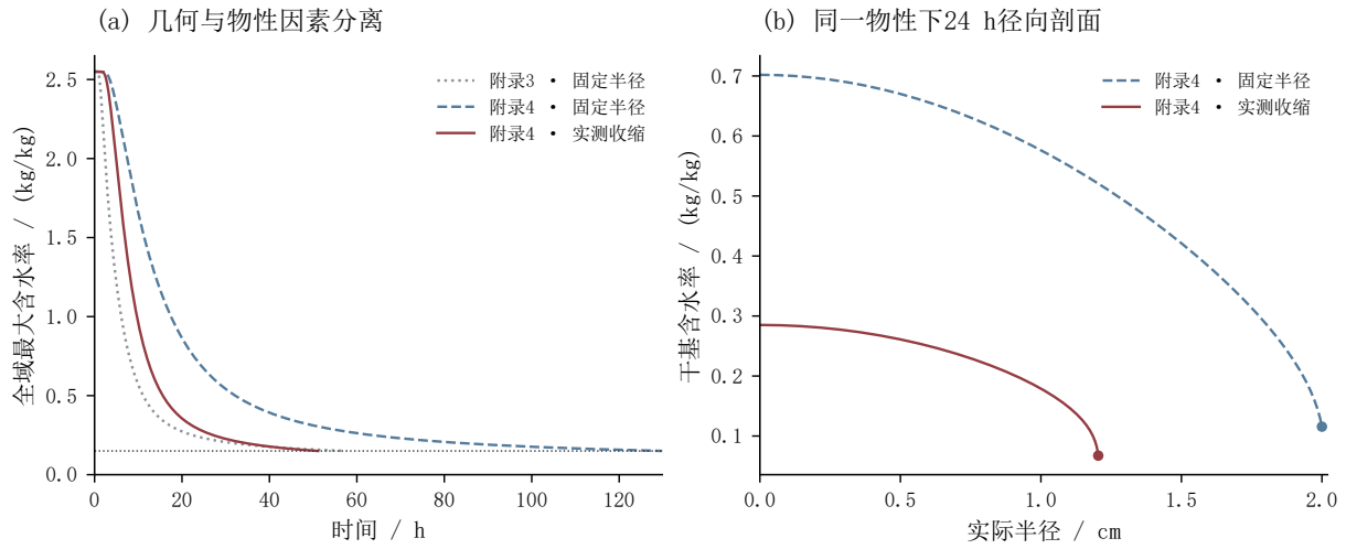
图 19 附录 4 下的收缩对照及与问题 3 的区别
