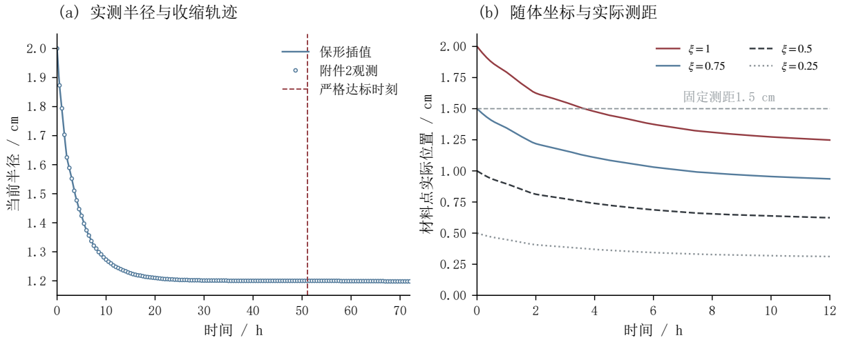
图 16 实测收缩与随体径向坐标
