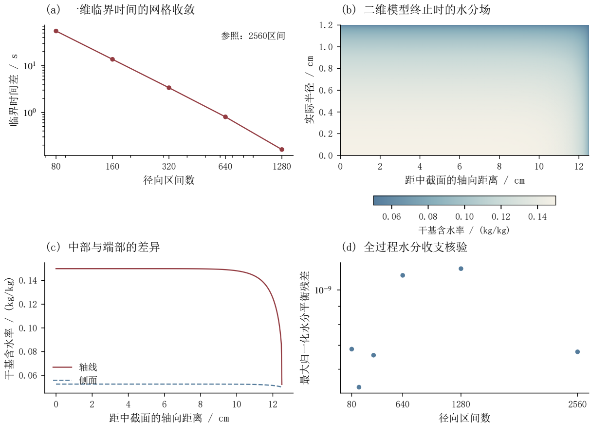
图 20 网格收敛、二维端部差异及水分收支检验
