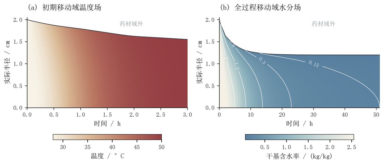
图 17 收缩域内的温度与干基含水率演化
