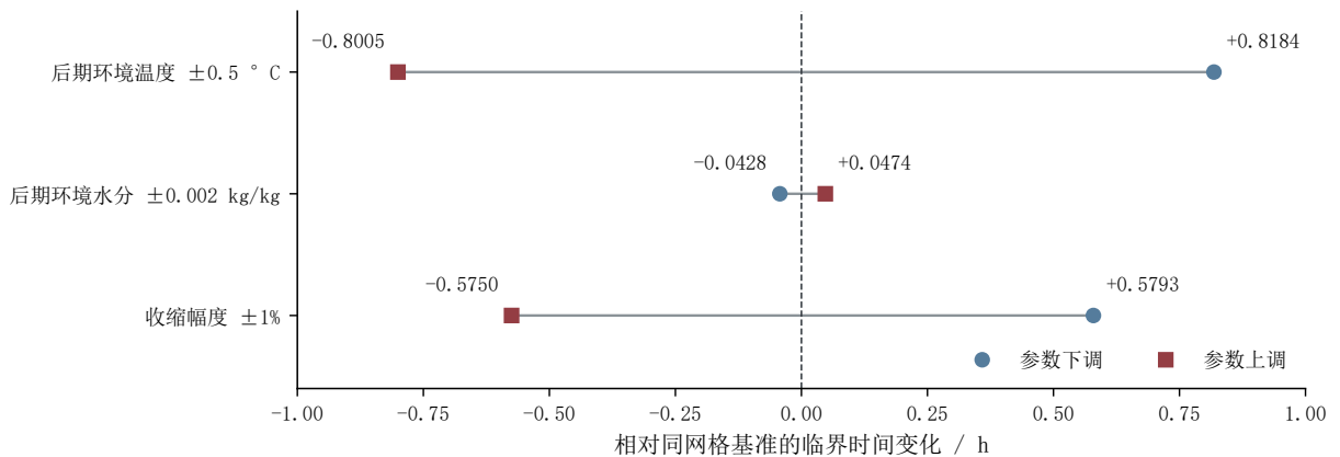
图 21 后期环境与收缩幅度对临界时间的影响
