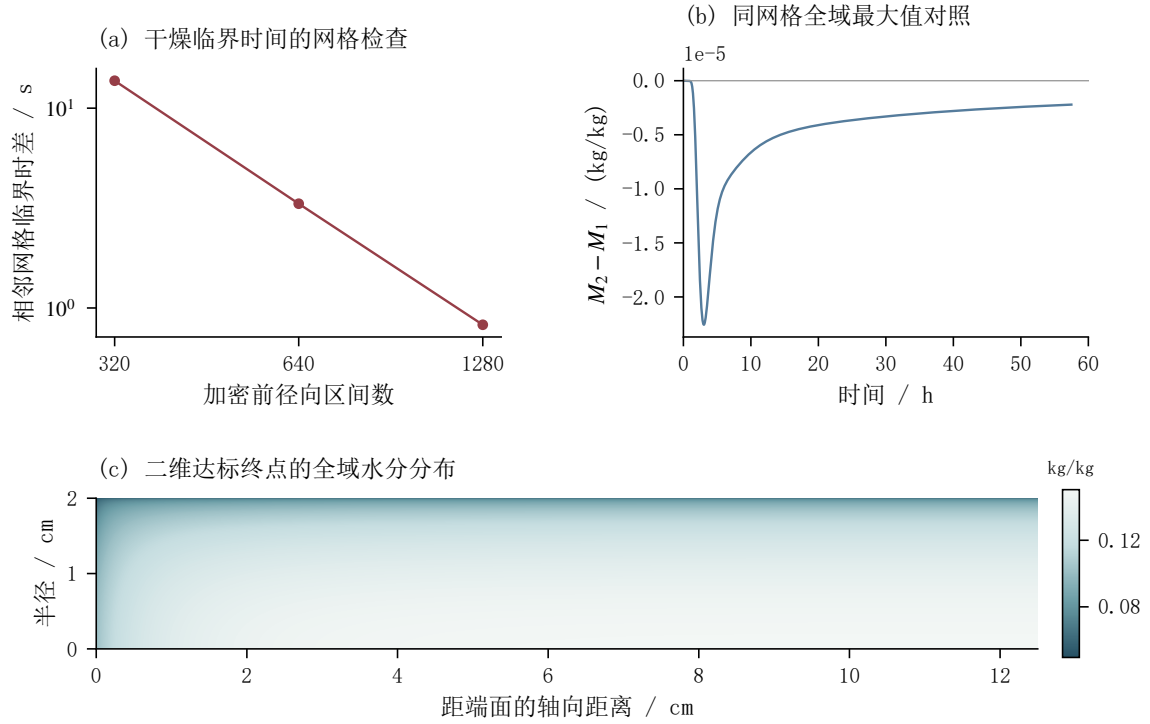
图 15 终止时间的数值与维度检验
