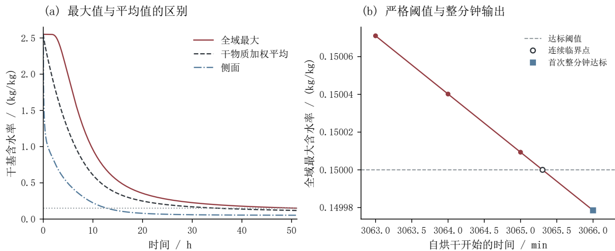
图 18 全域达标判据及终止时刻的局部核验
