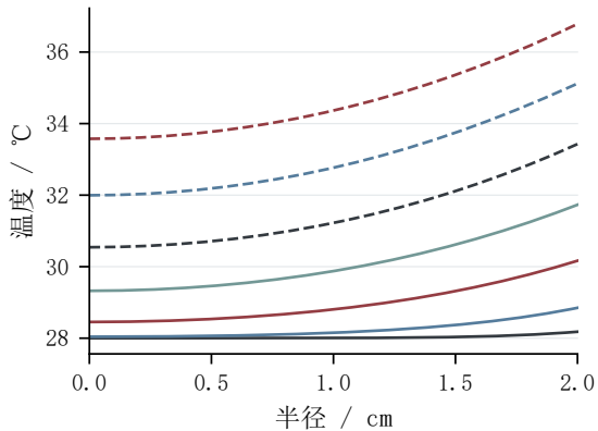
(a) 径向温度梯度
