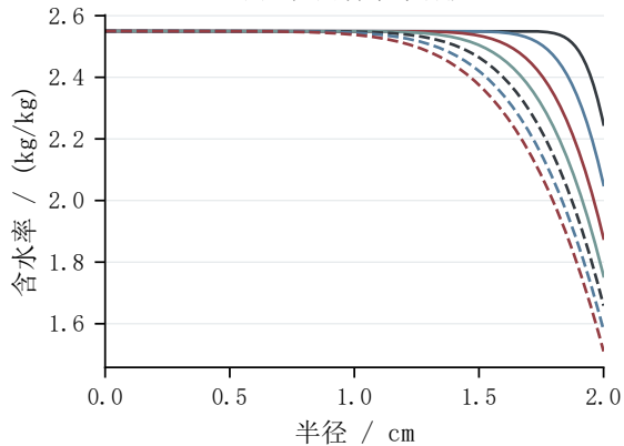
(b) 径向含水率梯度
