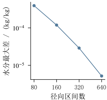
(b) 径向水分收敛
