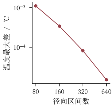
(a) 径向温度收敛
