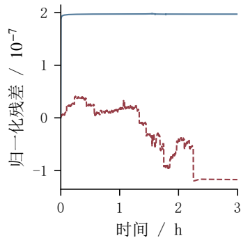
(c) 一维主解总体平衡
