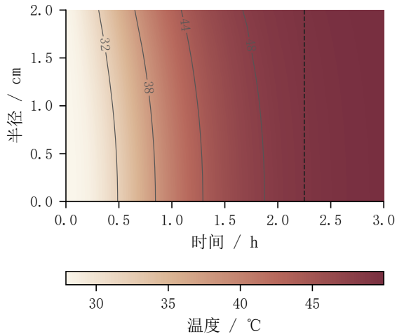
(a) 一维主解温度场
