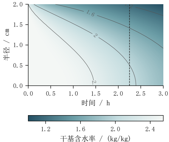
(b) 一维主解水分场
