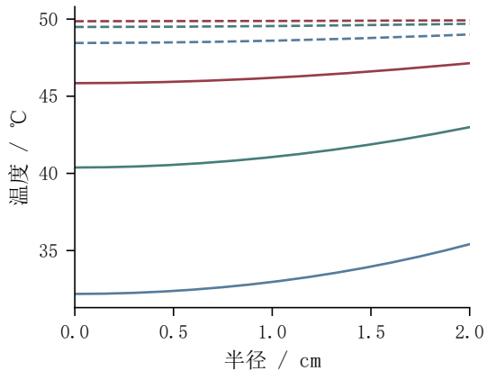
(a) 温度径向剖面
