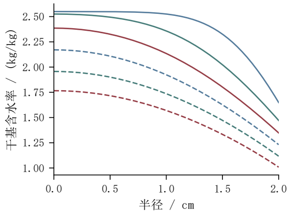
(b) 水分径向剖面
