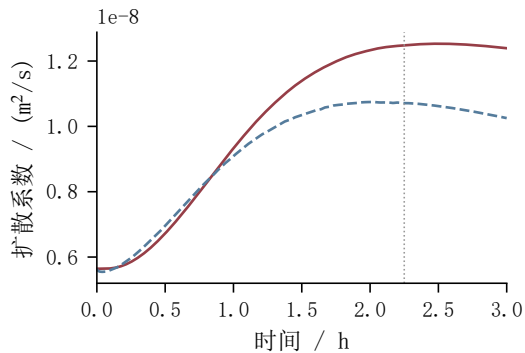
(d) 水分扩散系数
