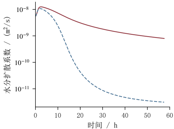
(a) 失水使后期扩散减慢
