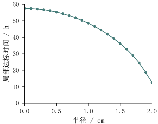
(b) 不同半径的达标次序
