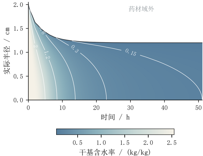
(b) 全过程移动域水分场
