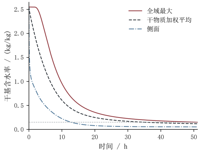
(a) 最大值与平均值的区别
