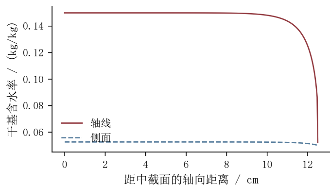
(c) 中部与端部的差异
