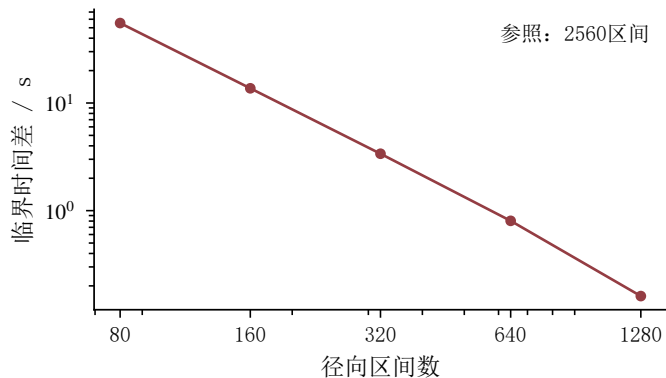
(a) 一维临界时间的网格收敛
