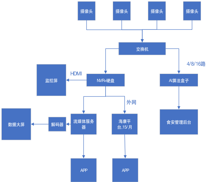
摄像头结构图
