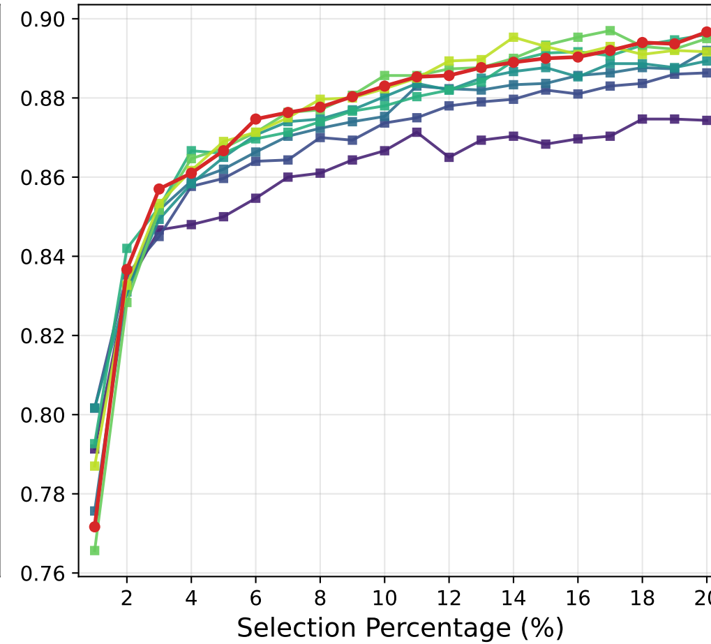
AG News
