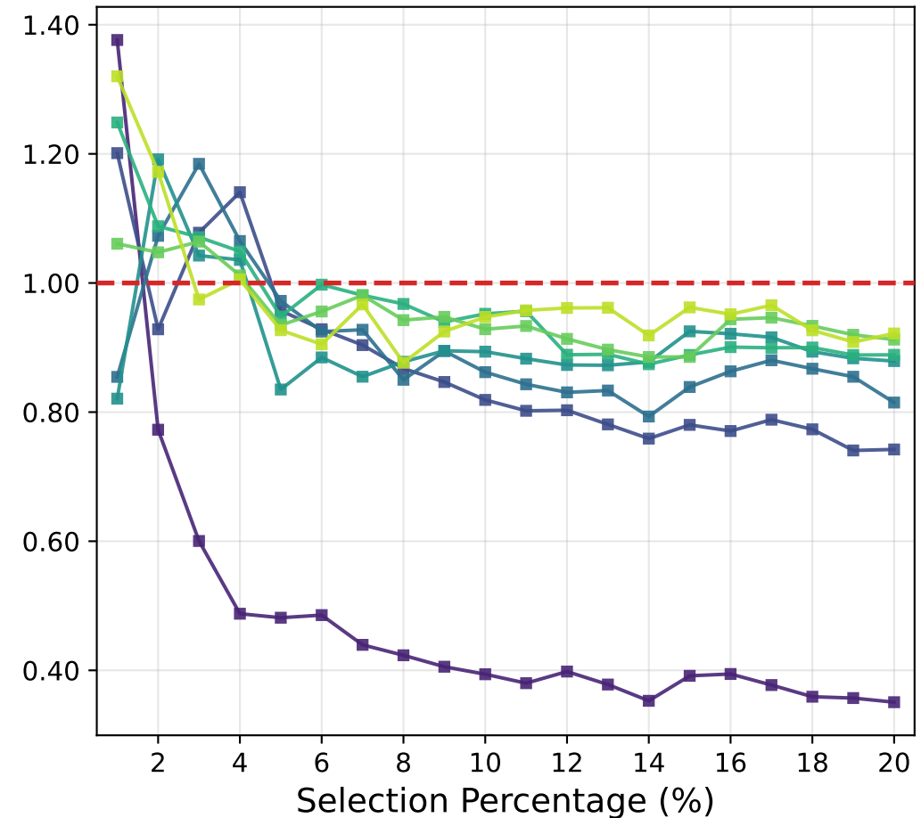
RTE ( n = 2490 )
